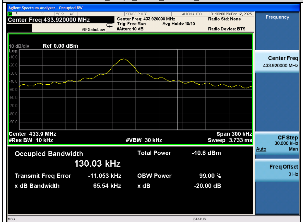
Test_Graph_GFSK_433.92MHz_OBW
