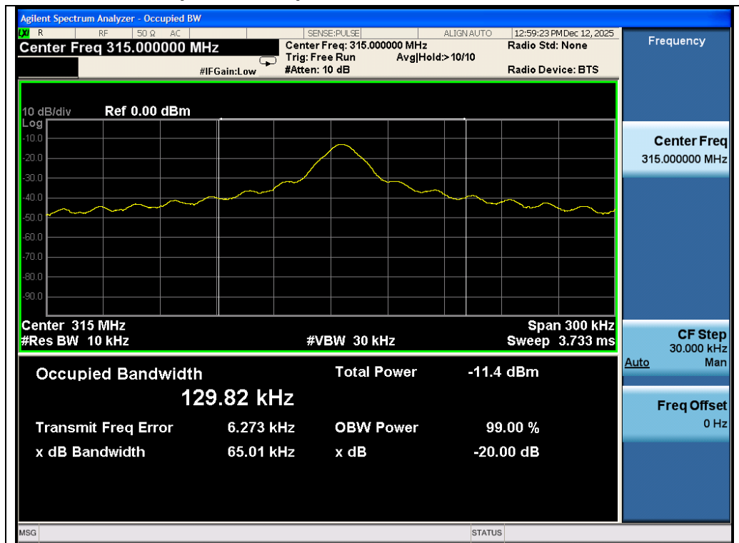
Test_Graph_GFSK_315MHz_OBW
