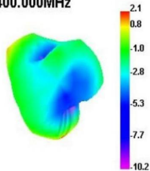
2400.000MHz
