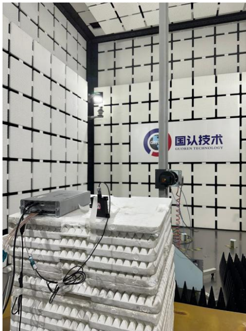
Fig.2(130-200GHZ)
