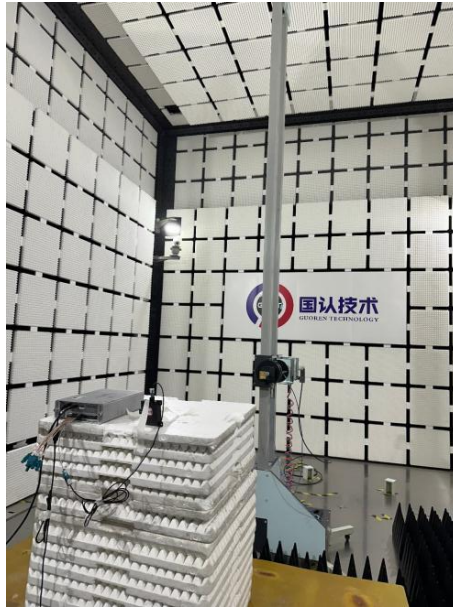
Fig.6(18-42GHZ)
