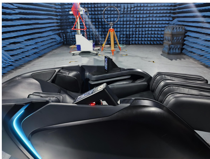
9K-30MHz
