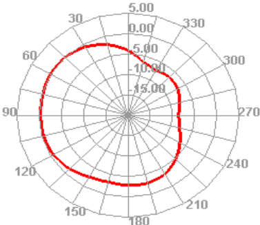
2400.000MHz H
