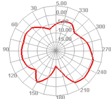
2500.000MHz E1
