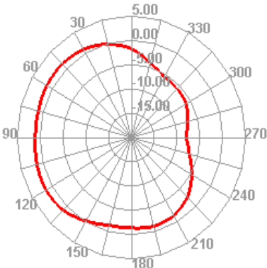
2500.000MHz H
