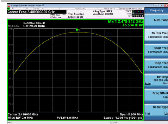
DH5-Ant4-2480-PASS
