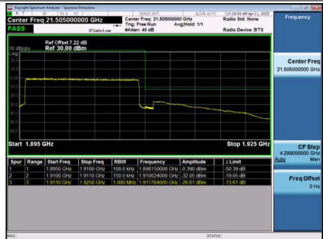
Band2-20MHz-QPSK-18700-100RB#0-PASS
