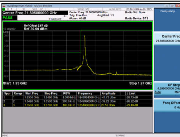
Band25-20MHz-QPSK-26140-1RB#0-PASS
