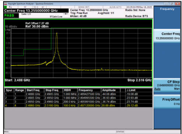
Band41-20MHz-QPSK-41490-1RB#99-PASS
