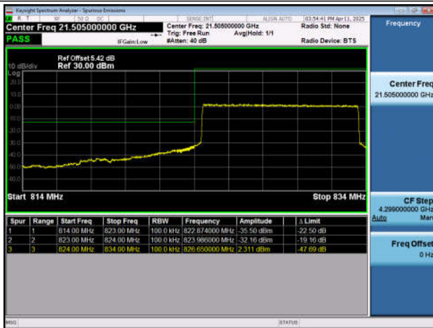
Band26(824-849)-10MHz-QPSK-26990-50RB#0-PASS
