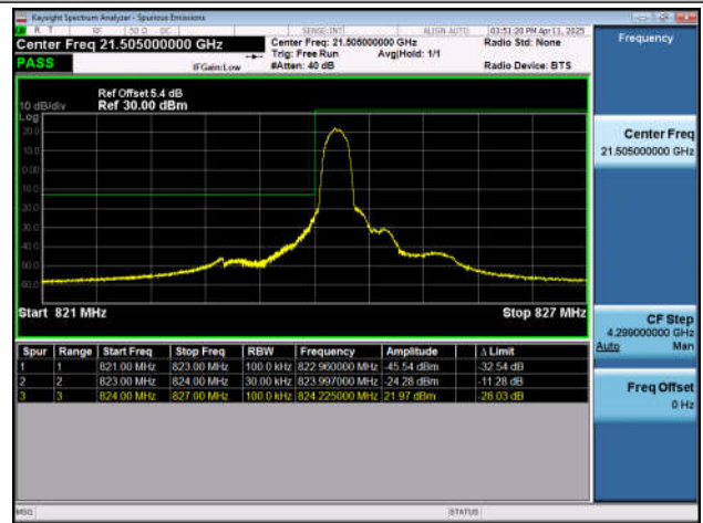
Band26(824-849)-3MHz-QPSK-27025-1RB#14-PASS
