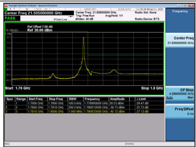
Band66-20MHz-QPSK-132572-1RB#99-PASS
