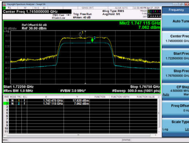
NTNT-n66-PC3-15-20-M-CP-256QAM-Outet_Full-Ant1-PA
