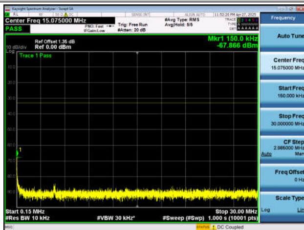
NTNV-n66-PC3-15-20-L-DFT-BPSK-Inner_1RB_Left-0.15-3 0-PASS
