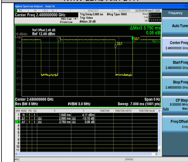
NTNV-2DH5-Ant4-2480
