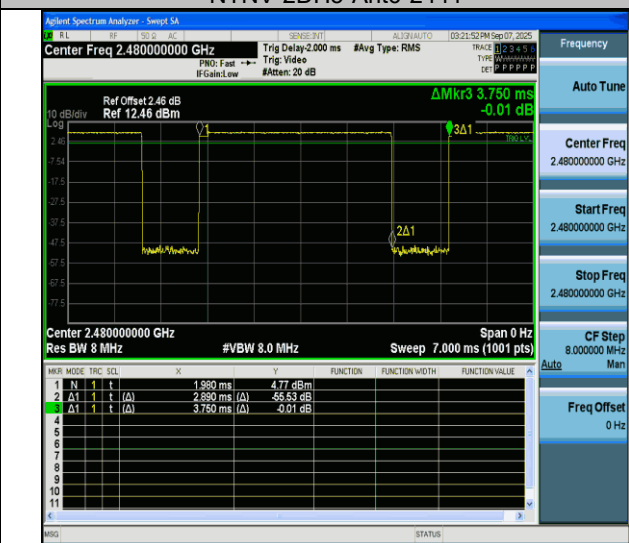
NTNV-2DH5-Ant6-2480
