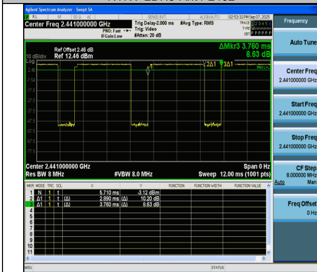
NTNV-2DH5-Ant4-2441
