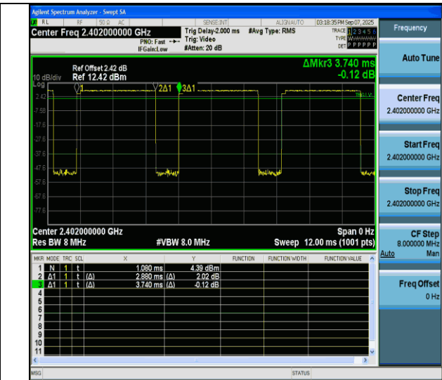
NTNV-2DH5-Ant6-2402
