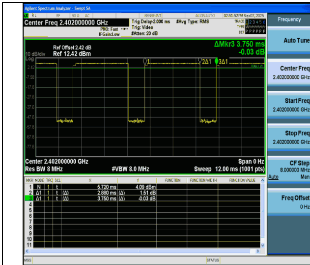
NTNV-2DH5-Ant4-2402
