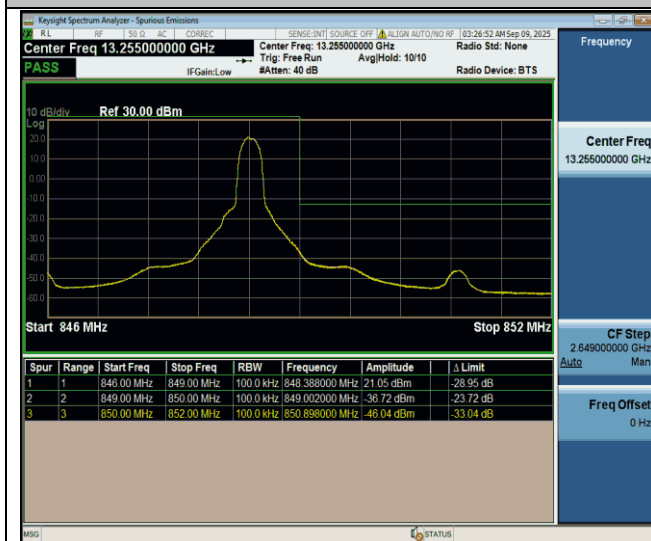
Band26(824-849)-10MHz-QPSK-26990-1RB#49-PASS
