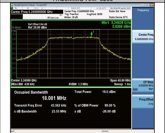
11n20MIMO-Ant7-5240
