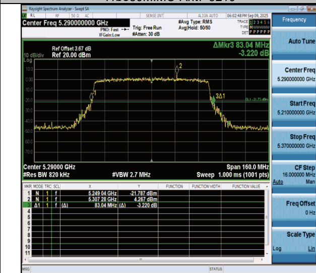
11be80MIMO-Ant7-5290
