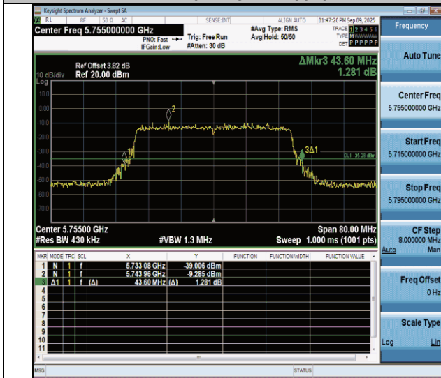
11ax40MIMO-Ant4-5755
