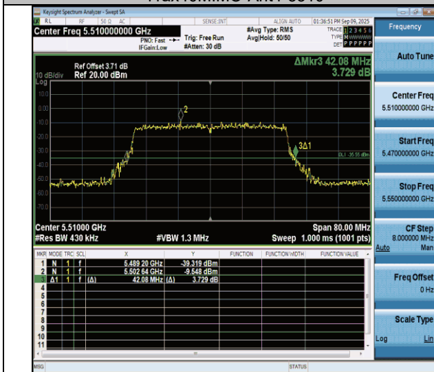
11ax40MIMO-Ant4-5510
