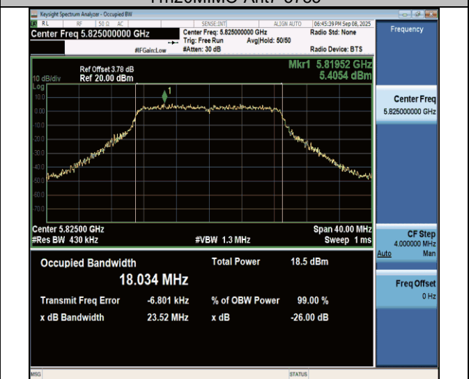
11n20MIMO-Ant7-5825
