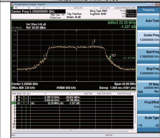
11ax20MIMO-Ant7-5200
