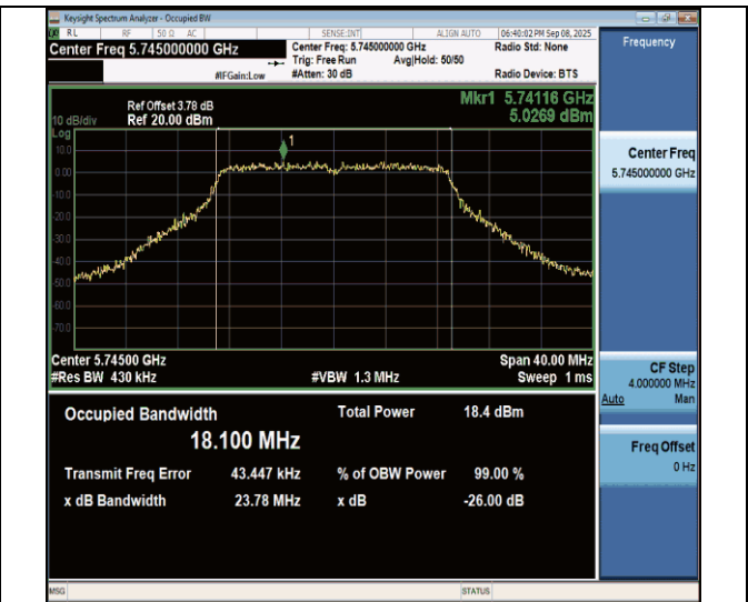
11n20MIMO-Ant7-5745
