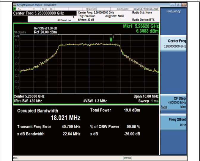
11n20MIMO-Ant7-5260
