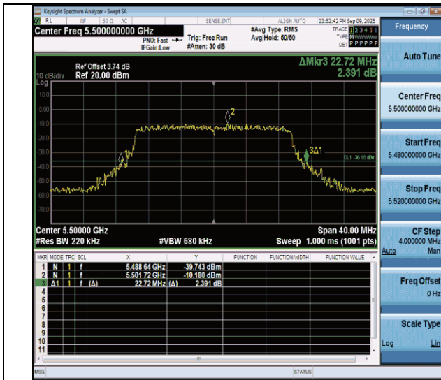
11be20MIMO-Ant4-5500
