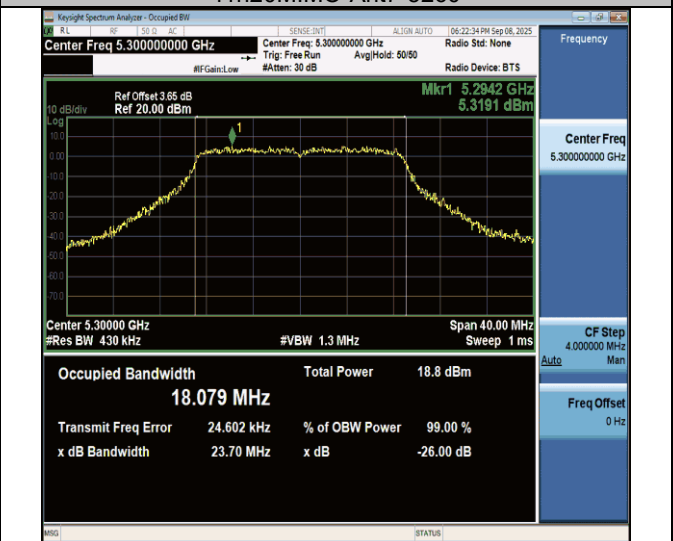
11n20MIMO-Ant7-5300
