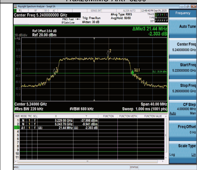
11ax20MIMO-Ant7-5240
