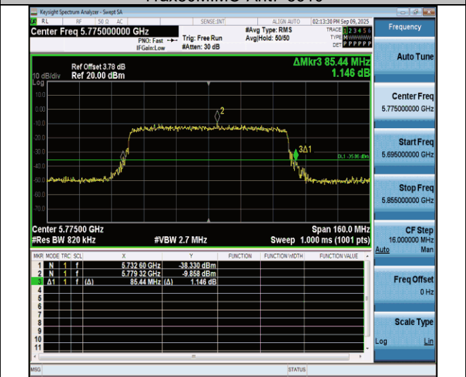
11ax80MIMO-Ant7-5775
