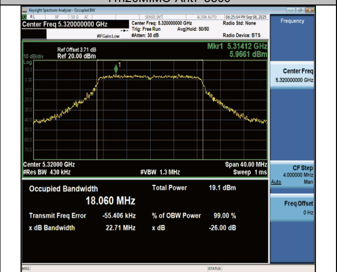
11n20MIMO-Ant7-5320
