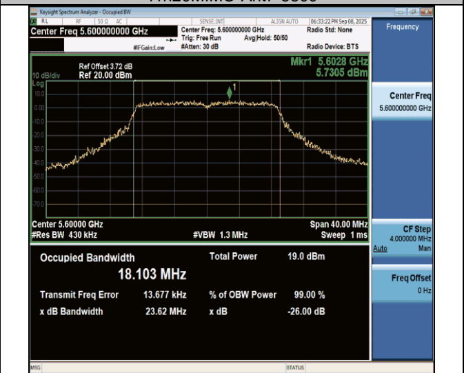
11n20MIMO-Ant7-5600
