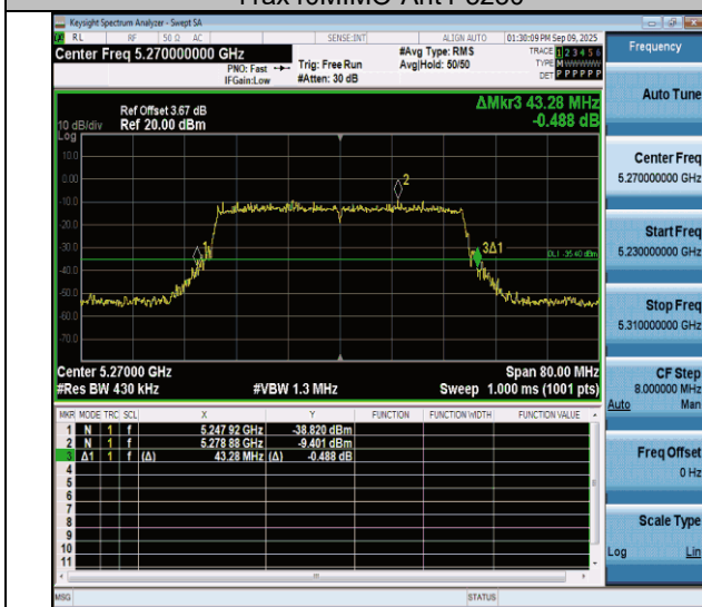
11ax40MIMO-Ant4-5270
