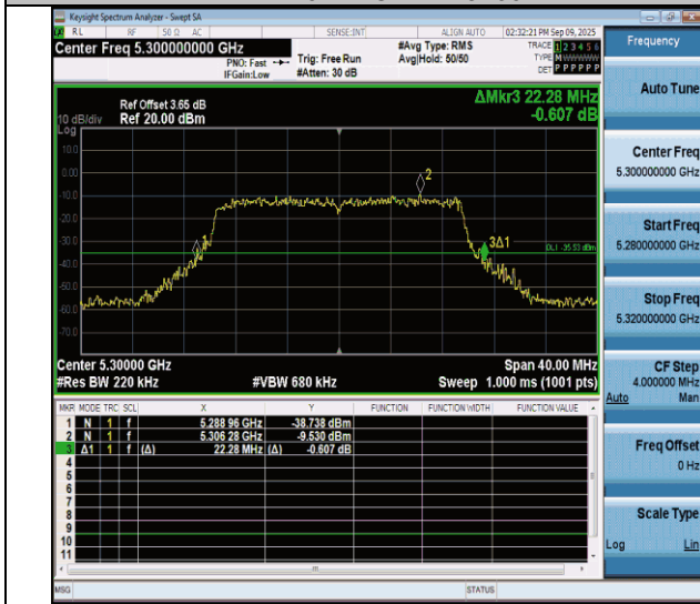
11be20MIMO-Ant4-5300
