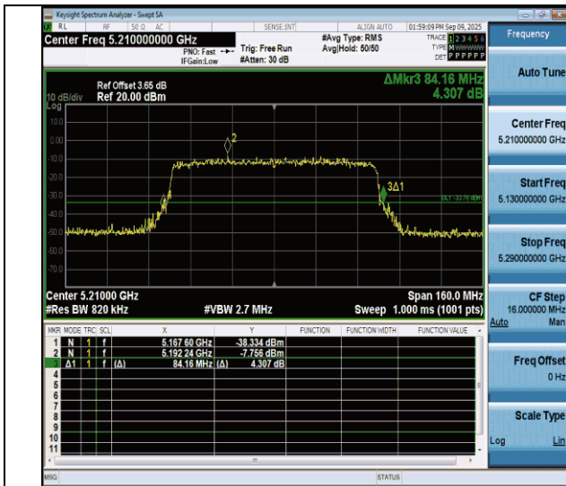
11ax80MIMO-Ant4-5210
