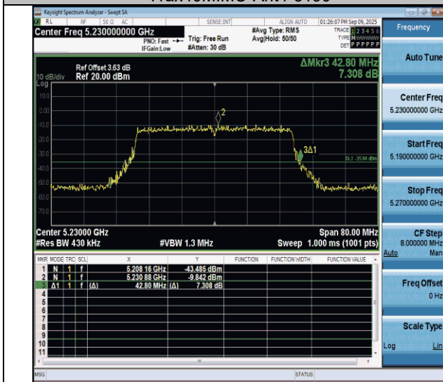
11ax40MIMO-Ant4-5230
