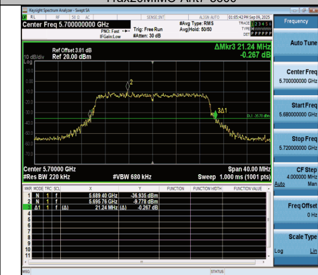
11ax20MIMO-Ant7-5700
