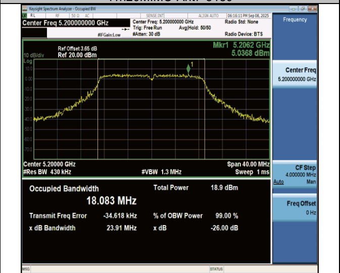
11n20MIMO-Ant7-5200
