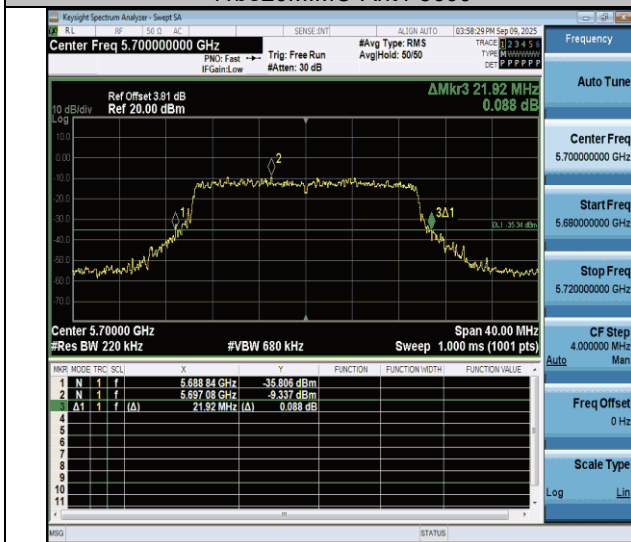
11be20MIMO-Ant4-5700
