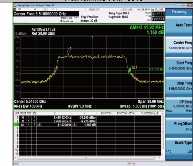
11ax40MIMO-Ant7-5510
