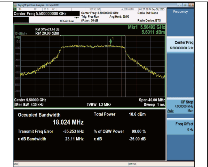
11n20MIMO-Ant7-5500
