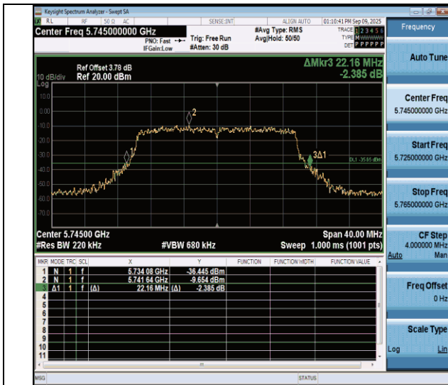
11ax20MIMO-Ant4-5745
