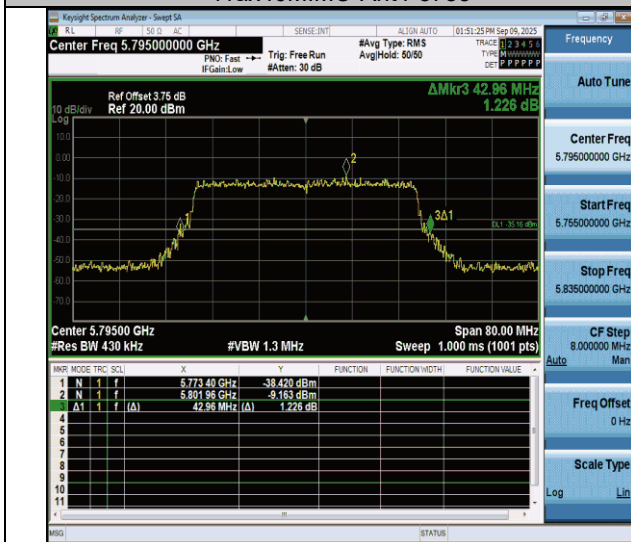
11ax40MIMO-Ant4-5795
