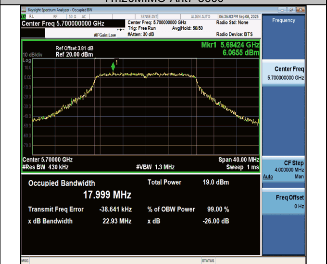
11n20MIMO-Ant7-5700
