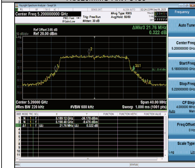
11be20MIMO-Ant4-5200
