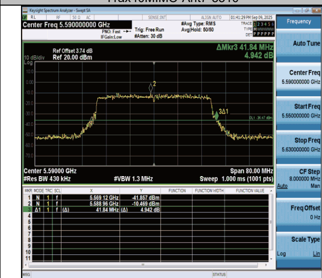
11ax40MIMO-Ant7-5590
