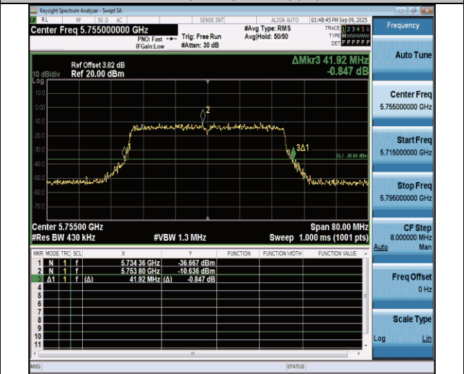
11ax40MIMO-Ant7-5755
