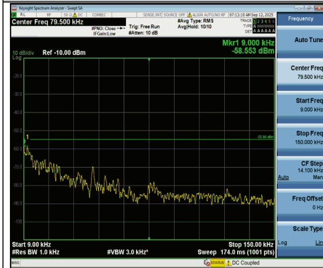
41-41-20MHz-20MHz-QPSK-QPSK-41292-41490-1RB#0-0RB#0- 0.009~0.15MHz-PASS
