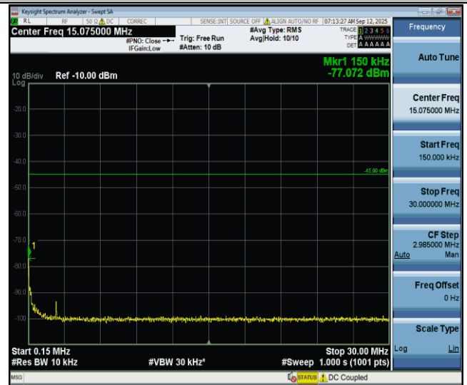
41-41-20MHz-20MHz-QPSK-QPSK-41292-41490-1RB#0-0RB#0- 0.15~30MHz-PASS
