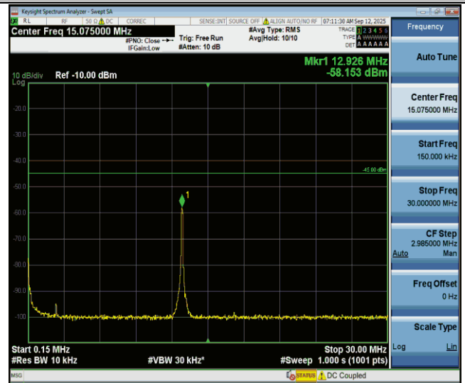
41-41-20MHz-20MHz-QPSK-QPSK-40521-40719-1RB#0-ORB#0- 0.15~30MHz-PASS
