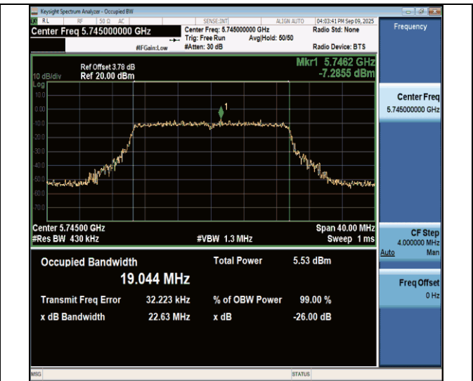
11be20MIMO-Ant7-5745
