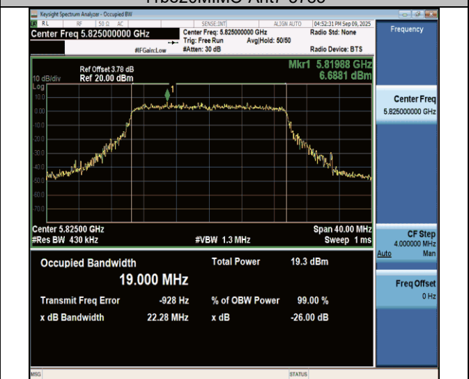
11be20MIMO-Ant7-5825
