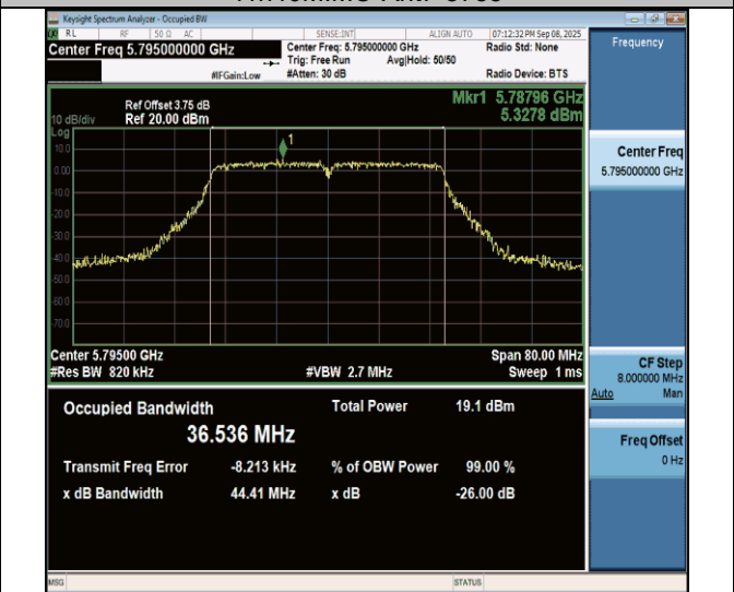
11n40MIMO-Ant7-5795
