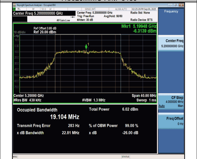
11be20MIMO-Ant7-5200
