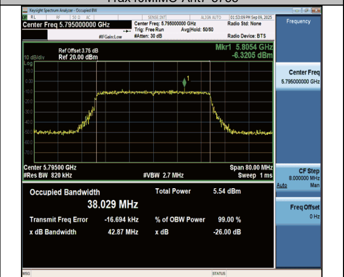
11ax40MIMO-Ant7-5795
