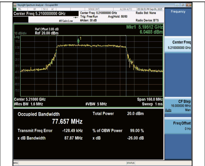
11be80MIMO-Ant7-5210
