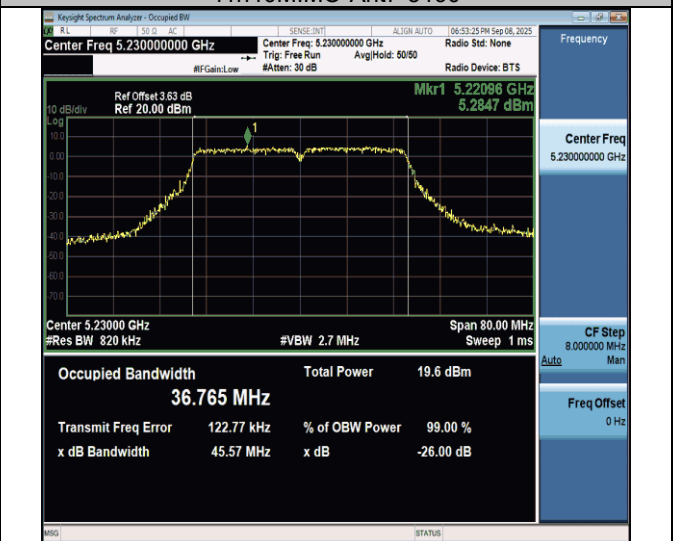
11n40MIMO-Ant7-5230
