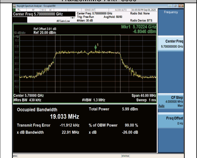
11ax20MIMO-Ant7-5700
