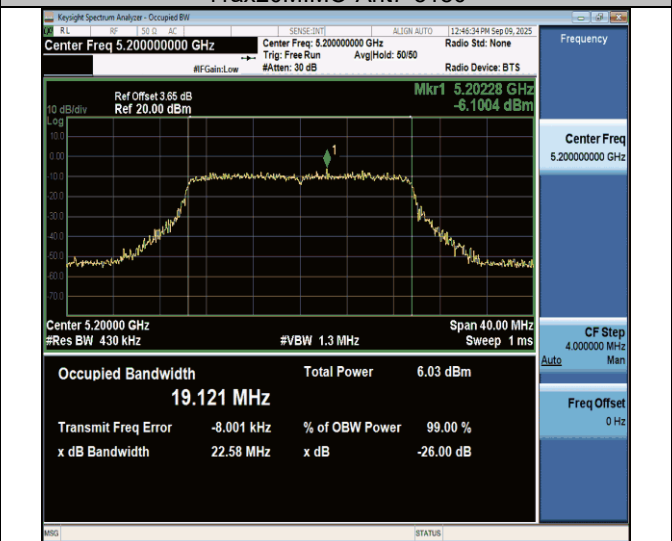
11ax20MIMO-Ant7-5200
