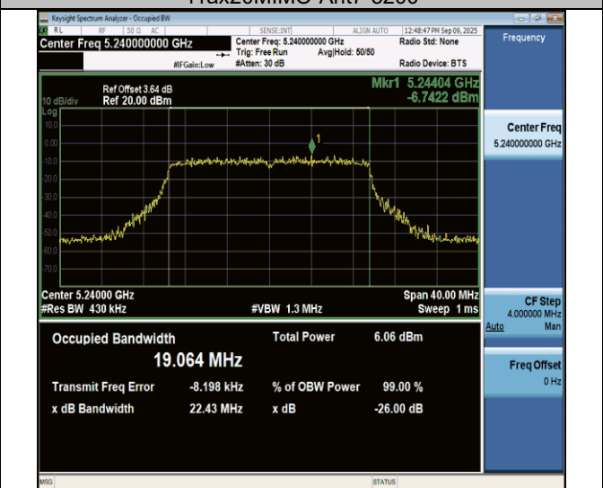
11ax20MIMO-Ant7-5240
