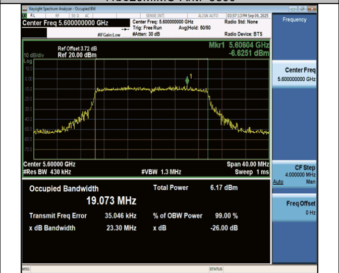
11be20MIMO-Ant7-5600
