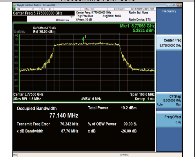
11be80MIMO-Ant7-5775
