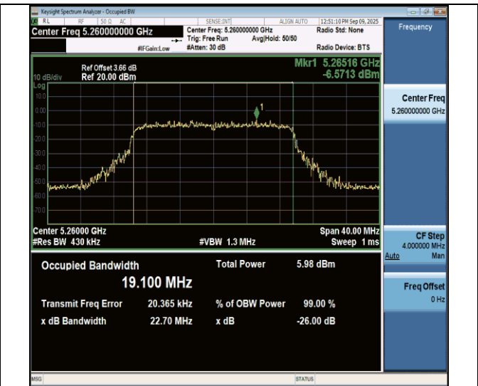
11ax20MIMO-Ant7-5260
