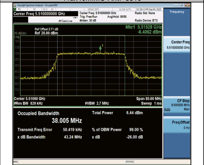
11ax40MIMO-Ant7-5510
