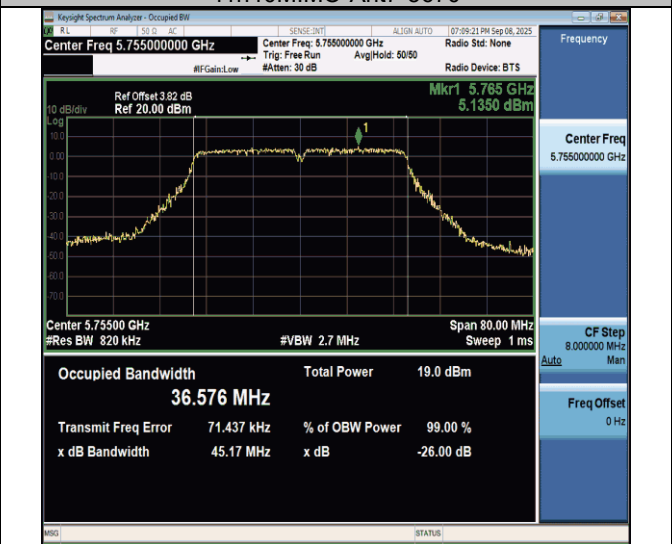
11n40MIMO-Ant7-5755
