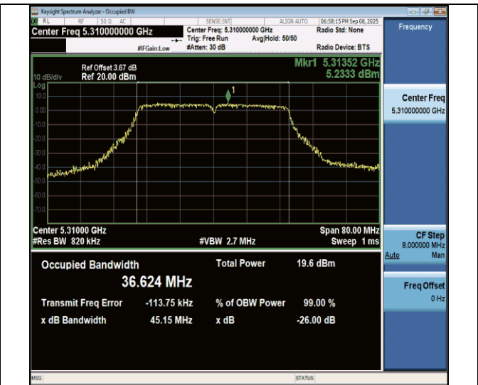
11n40MIMO-Ant7-5310
