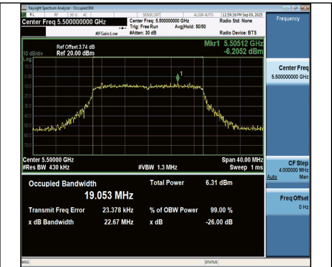
11ax20MIMO-Ant7-5500
