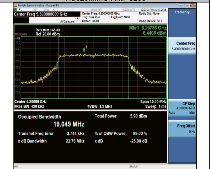
11be20MIMO-Ant7-5300
