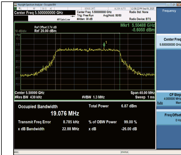
11ax20MIMO-Ant4-5500
