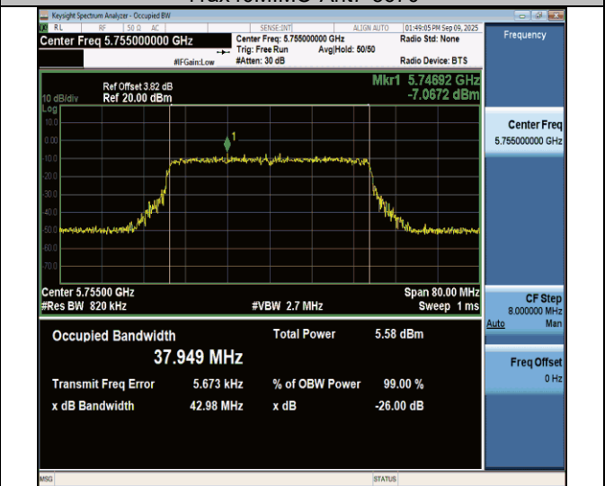
11ax40MIMO-Ant7-5755
