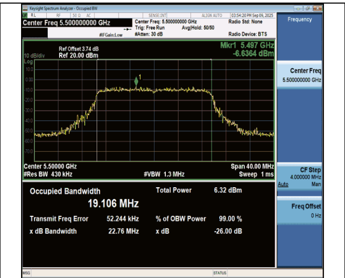
11be20MIMO-Ant7-5500
