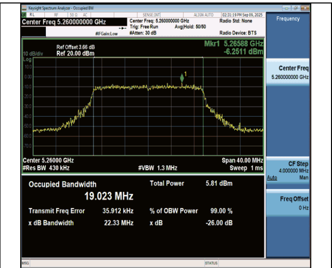
11be20MIMO-Ant7-5260
