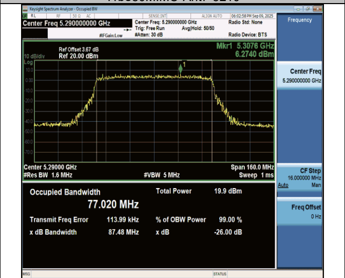
11be80MIMO-Ant7-5290
