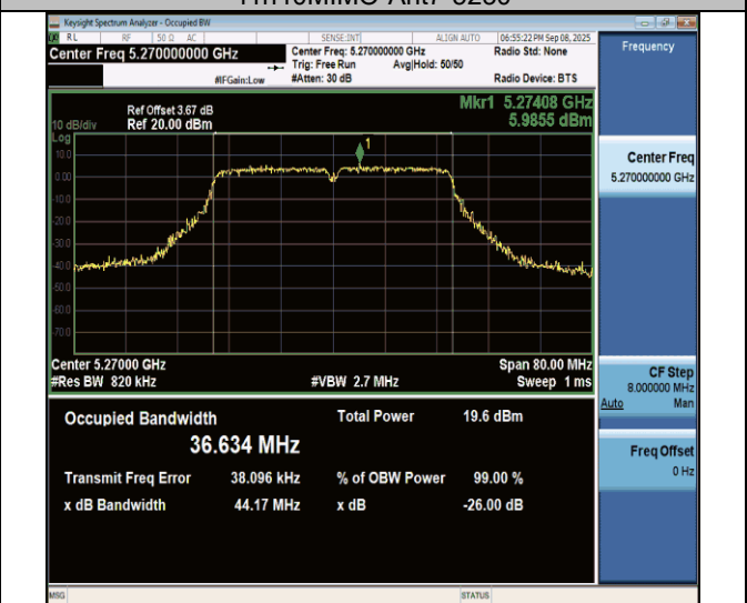
11n40MIMO-Ant7-5270
