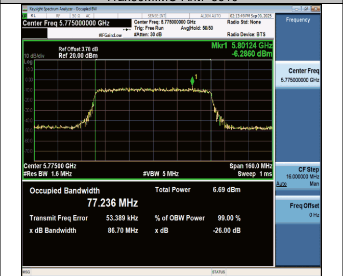
11ax80MIMO-Ant7-5775
