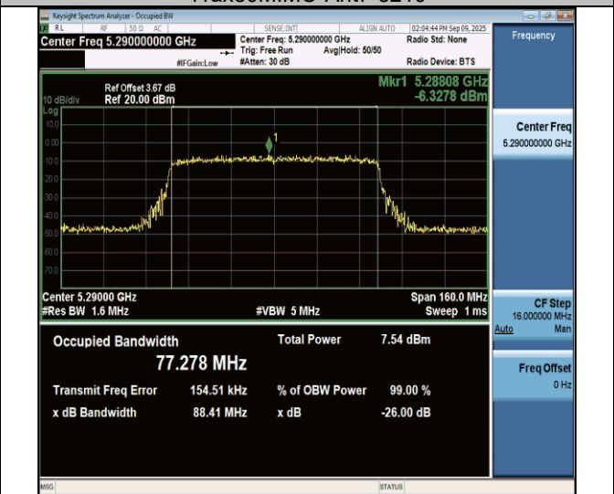
11ax80MIMO-Ant7-5290
