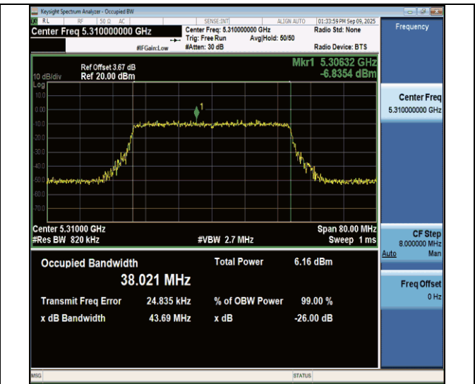
11ax40MIMO-Ant7-5310
