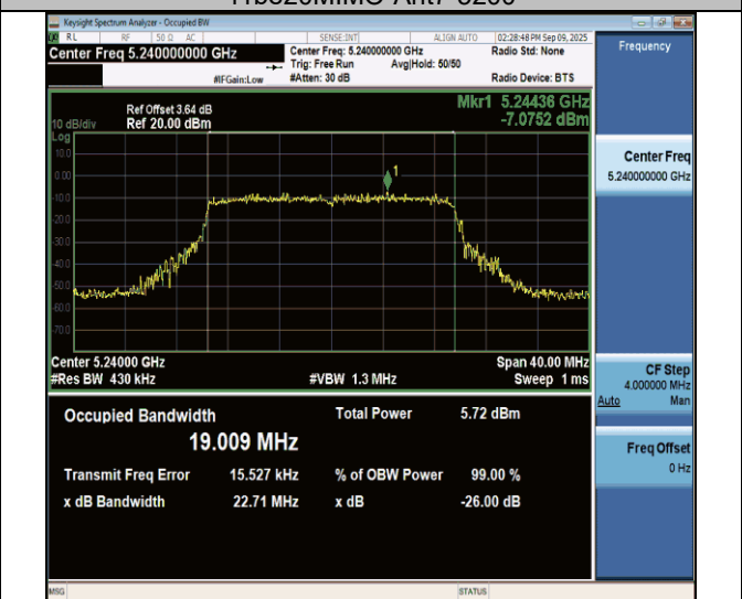
11be20MIMO-Ant7-5240
