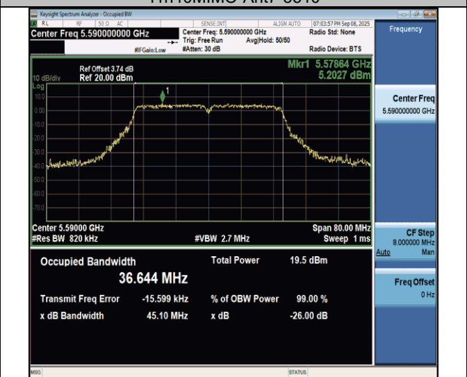
11n40MIMO-Ant7-5590
