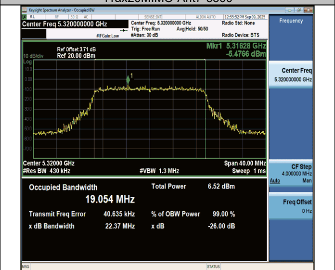
11ax20MIMO-Ant7-5320
