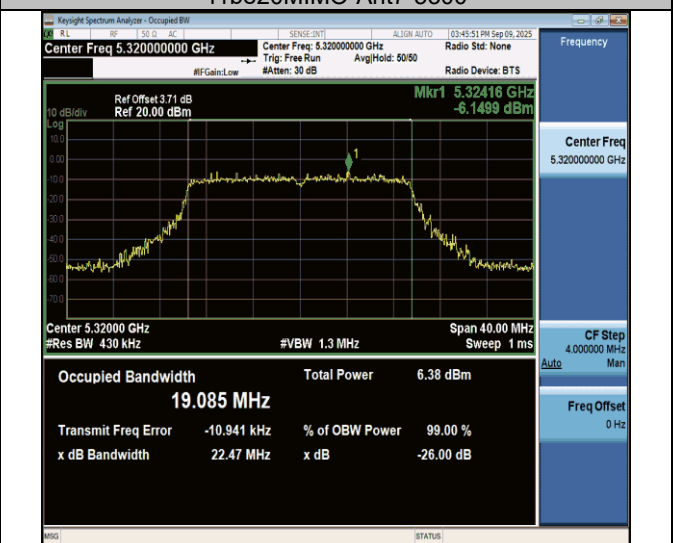
11be20MIMO-Ant7-5320
