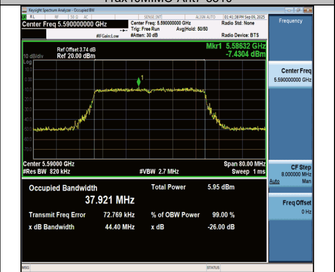
11ax40MIMO-Ant7-5590
