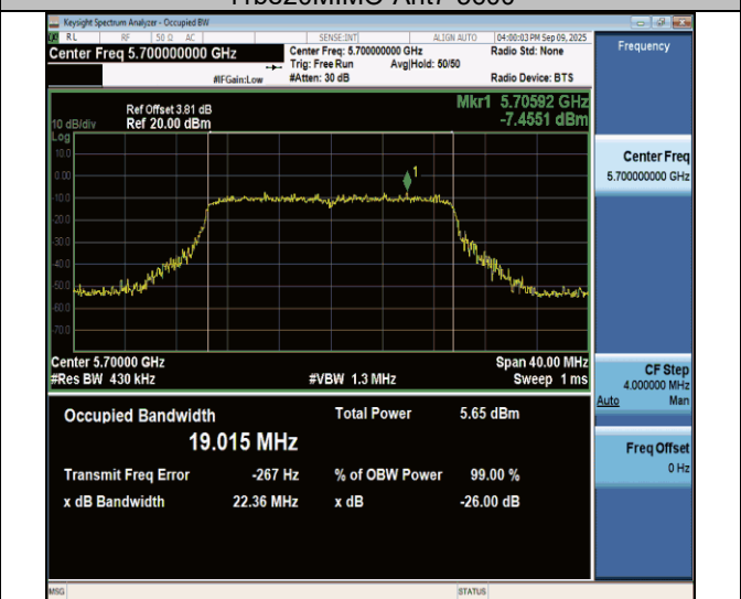
11be20MIMO-Ant7-5700
