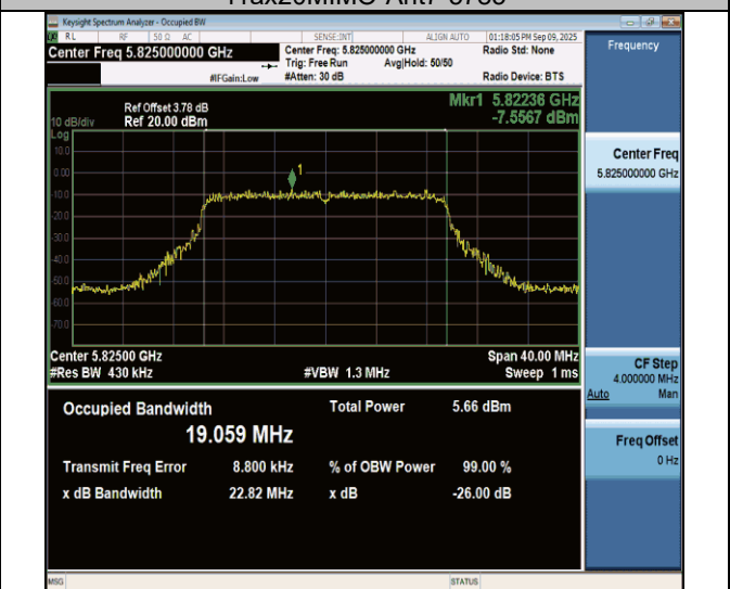
11ax20MIMO-Ant7-5825
