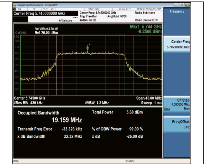
11ax20MIMO-Ant7-5745
