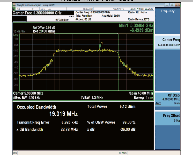
11ax20MIMO-Ant7-5300
