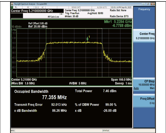
11ax80MIMO-Ant7-5210
