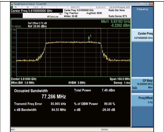
11ax80MIMO-Ant7-5610
