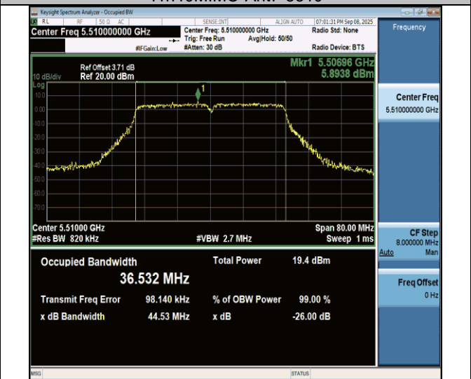
11n40MIMO-Ant7-5510
