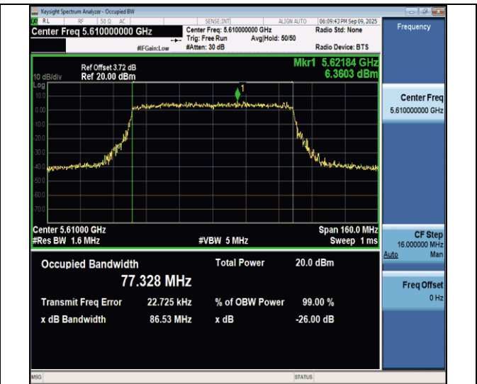
11be80MIMO-Ant7-5610
