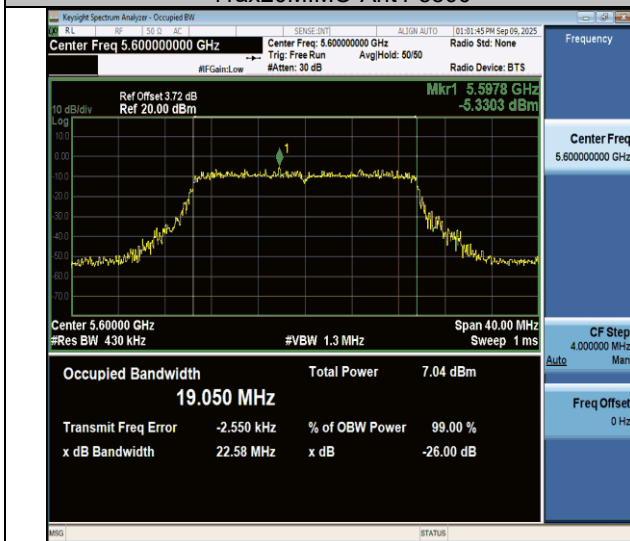
11ax20MIMO-Ant4-5600
