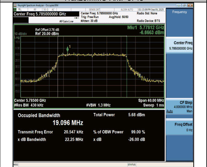
11ax20MIMO-Ant7-5785
