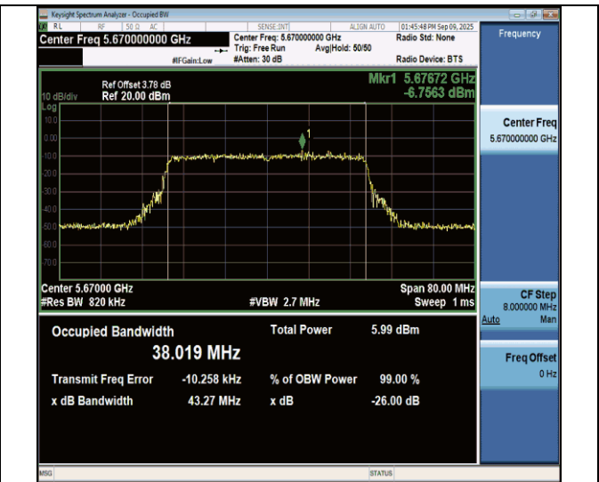
11ax40MIMO-Ant7-5670
