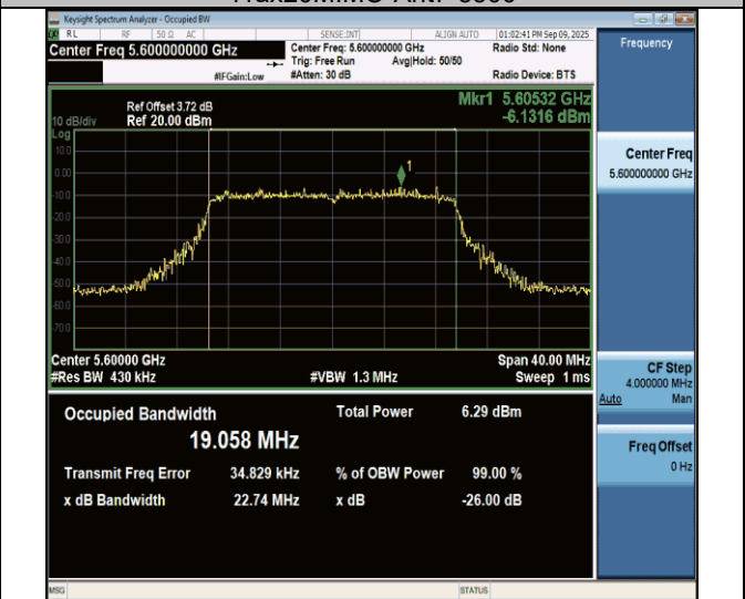
11ax20MIMO-Ant7-5600
