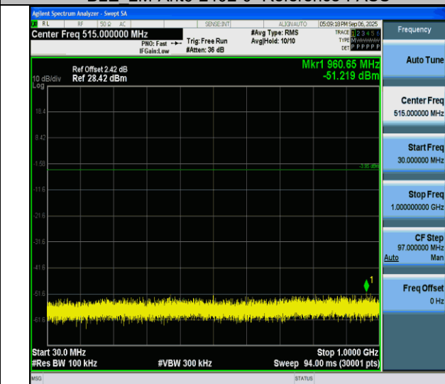
BLE 2M-Ant6-2402-30~1000-PASS
