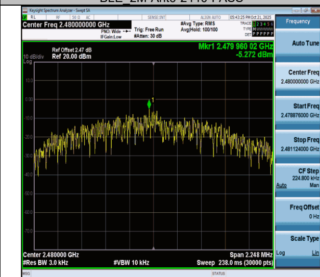
BLE 2M-Ant6-2480-PASS
