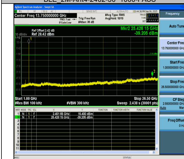
BLE 2M-Ant4-2402-1000~26500-PASS
