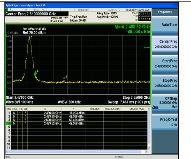
BLE 2M-Ant6-2480-PASS
