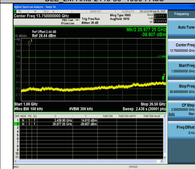
BLE 2M-Ant6-2440-1000~26500-PASS
