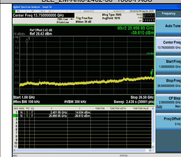
BLE 2M-Ant6-2402-1000~26500-PASS
