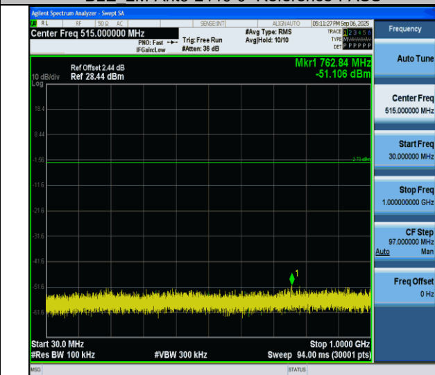
BLE 2M-Ant6-2440-30~1000-PASS
