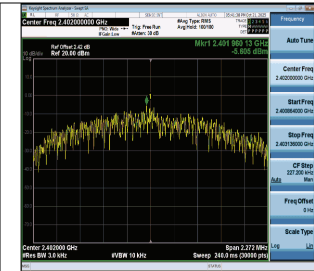
BLE 2M-Ant6-2402-PASS
