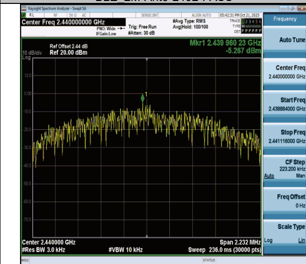
BLE 2M-Ant6-2440-PASS
