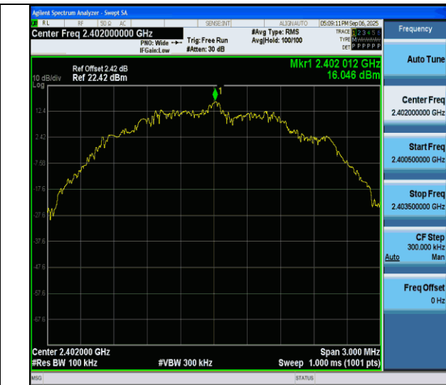
BLE 2M-Ant6-2402-0~Reference-PASS
