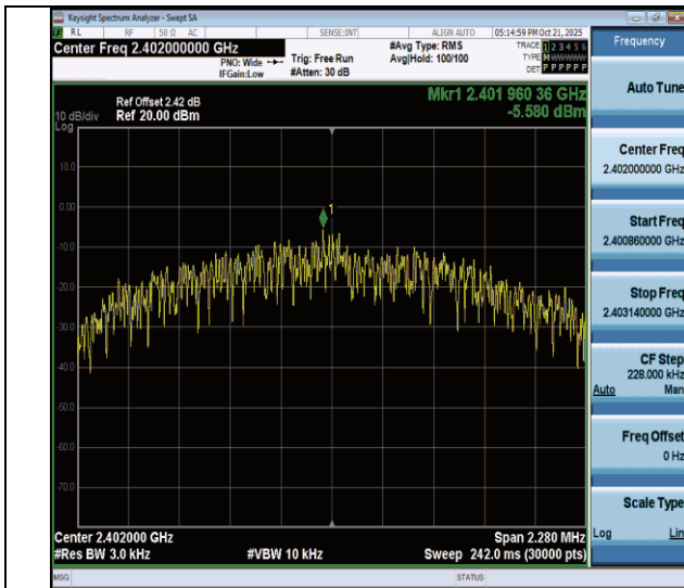
BLE 2M-Ant4-2402-PASS
