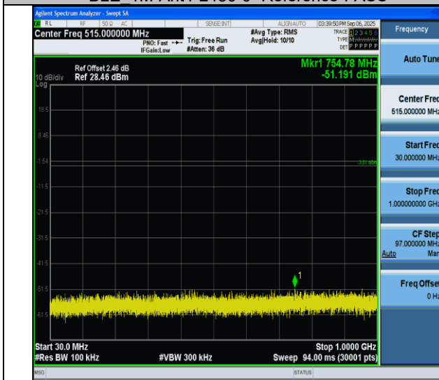
BLE 1M-Ant4-2480-30~1000-PASS
