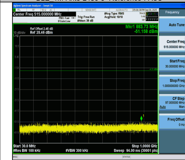
BLE 1M-Ant6-2480-30~1000-PASS
