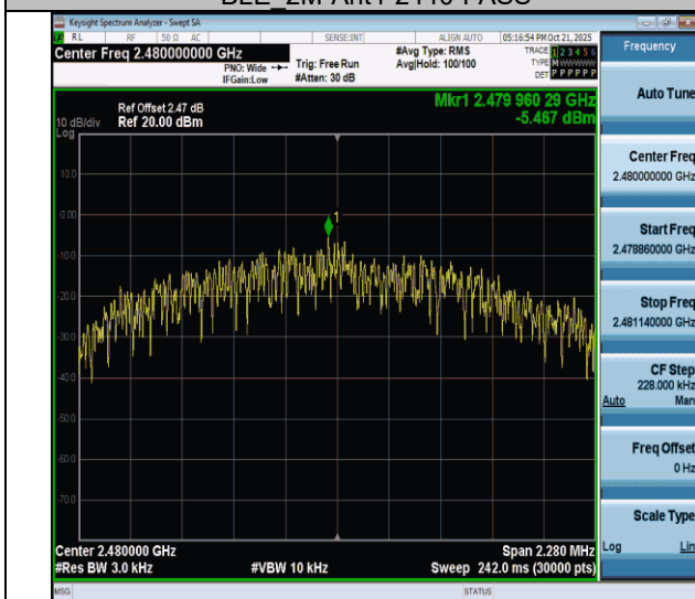
BLE 2M-Ant4-2480-PASS
