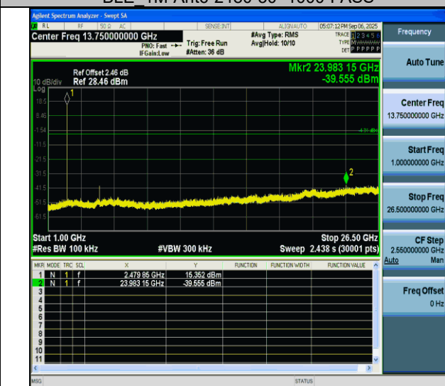
BLE 1M-Ant6-2480-1000~26500-PASS
