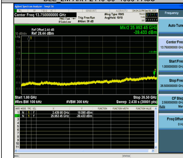
BLE 2M-Ant4-2440-1000~26500-PASS
