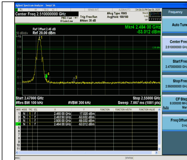
BLE 2M-Ant4-2480-PASS
