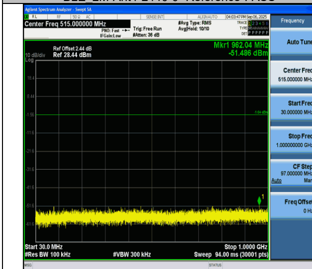
BLE 2M-Ant4-2440-30~1000-PASS
