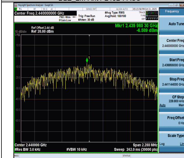
BLE 2M-Ant4-2440-PASS
