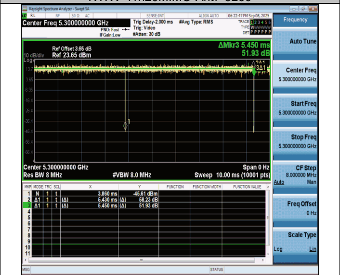
NTNV-11n20MIMO-Ant7-5300
