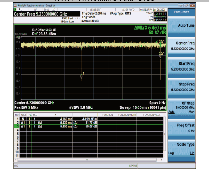
NTNV-11n40MIMO-Ant7-5230
