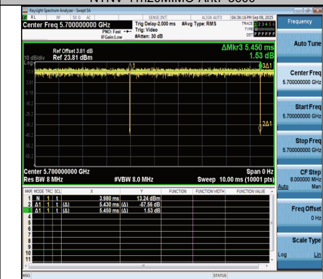
NTNV-11n20MIMO-Ant7-5700
