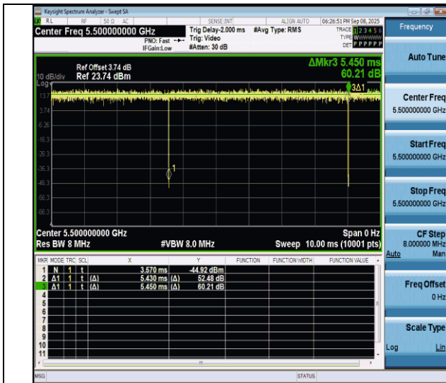
NTNV-11n20MIMO-Ant4-5500
