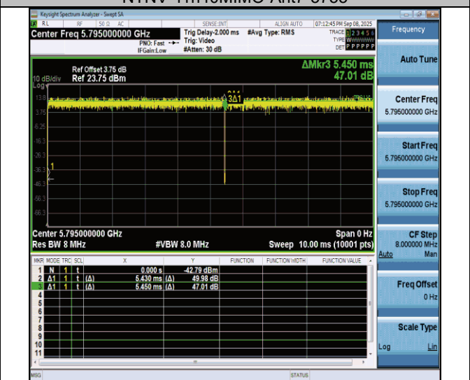
NTNV-11n40MIMO-Ant7-5795
