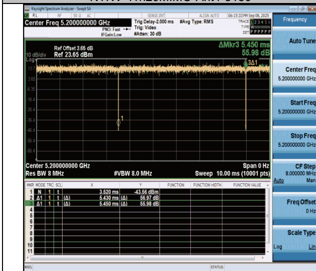
NTNV-11n20MIMO-Ant4-5200
