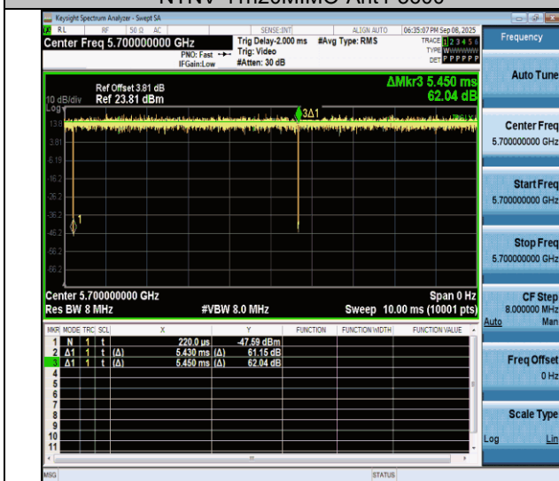
NTNV-11n20MIMO-Ant4-5700
