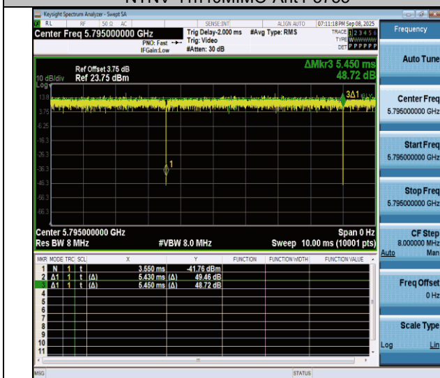
NTNV-11n40MIMO-Ant4-5795
