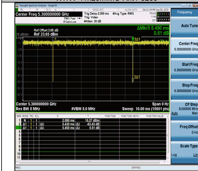
NTNV-11n20MIMO-Ant4-5300
