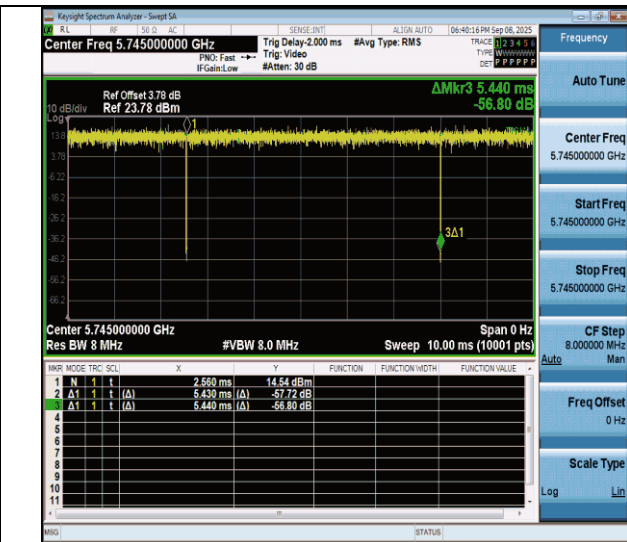
NTNV-11n20MIMO-Ant7-5745
