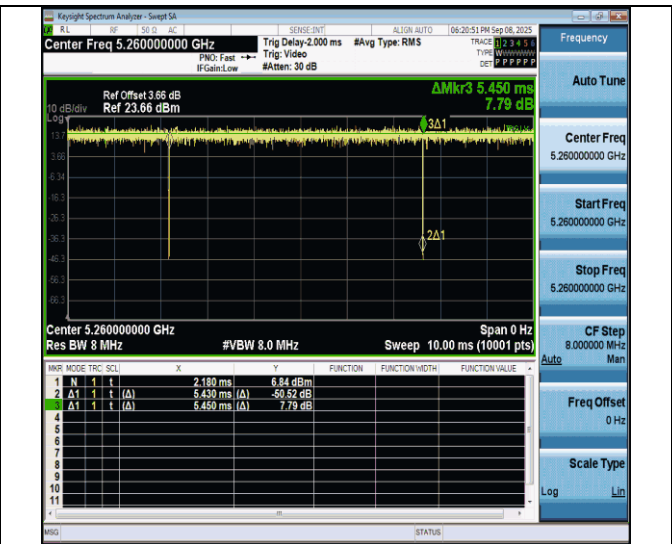
NTNV-11n20MIMO-Ant7-5260
