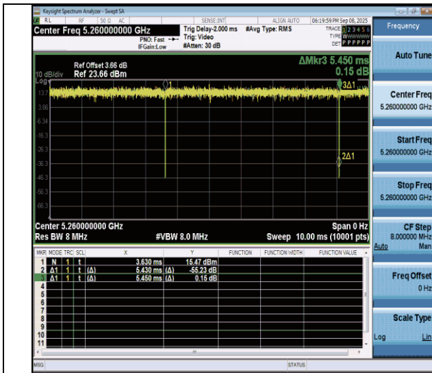
NTNV-11n20MIMO-Ant4-5260
