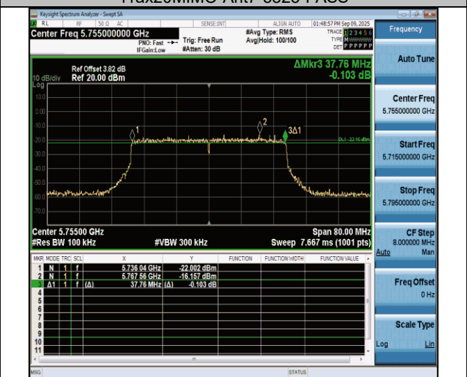
11ax40MIMO-Ant7-5755-PASS
