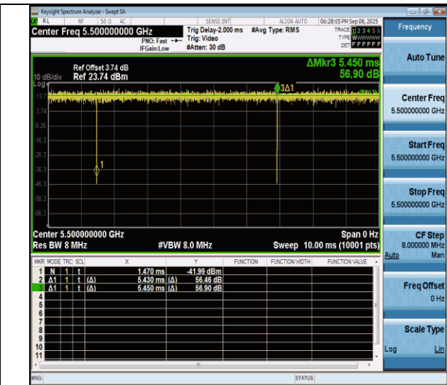
NTNV-11n20MIMO-Ant7-5500
