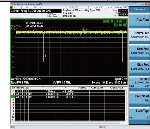
NTNV-11n20MIMO-Ant7-5200
