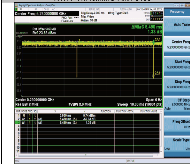
NTNV-11n40MIMO-Ant4-5230
