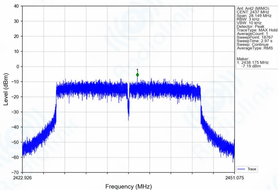
802.11ax(HEW20)_MCH_2437MHz_SU / MIMO_NTNV
