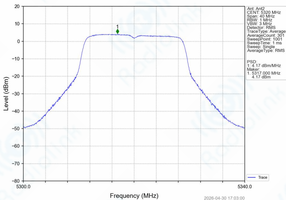
802.11n(HT20)_HCH_5320MHz_MIMO_NTNV
