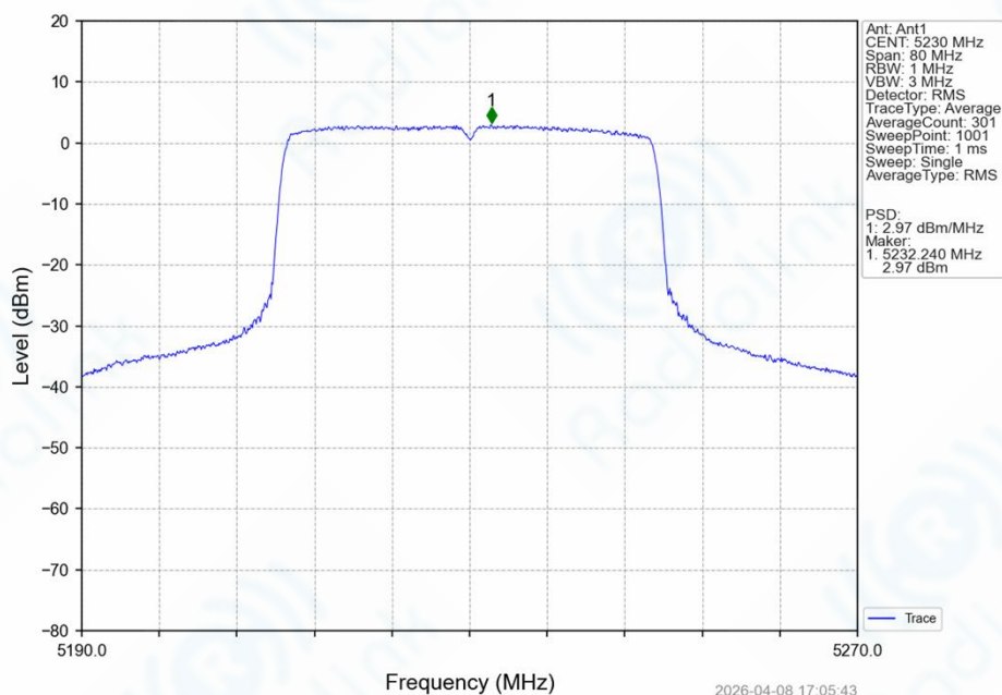
802.11ax(HEW40)_HCH_5230MHz_SU / _Ant1_NTNV
