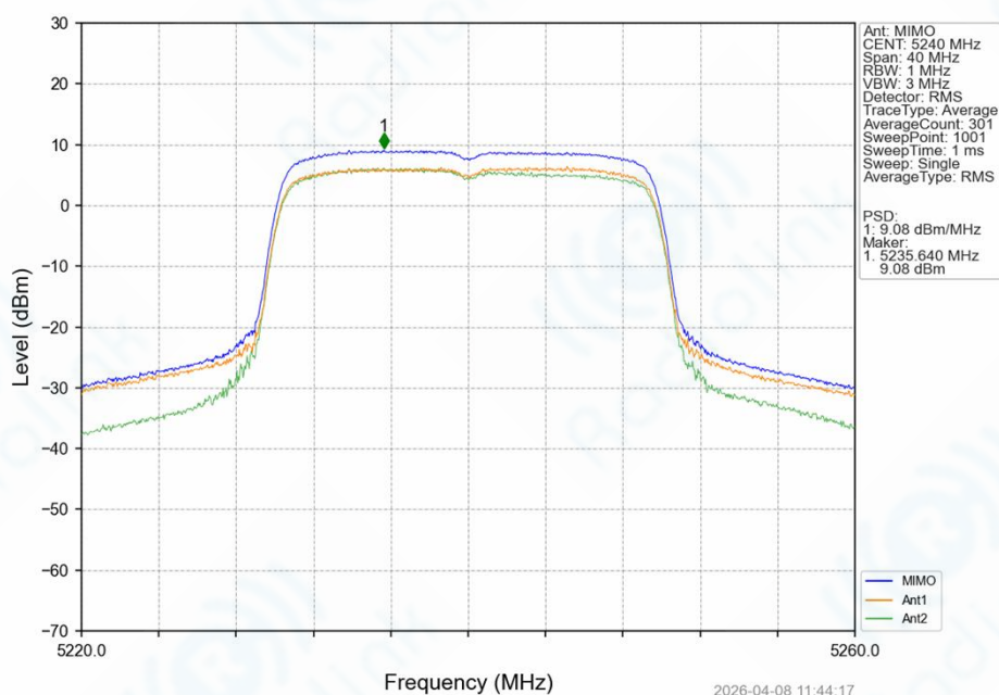
802.11ax(HEW20) HCH 5240MHz SU / MIMO NTN
