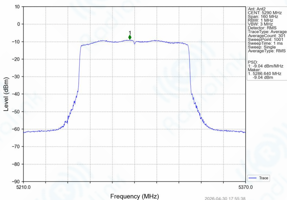
802.11ax(HEW80)_MCH_5290MHz_SU / _Ant2_NTNV
