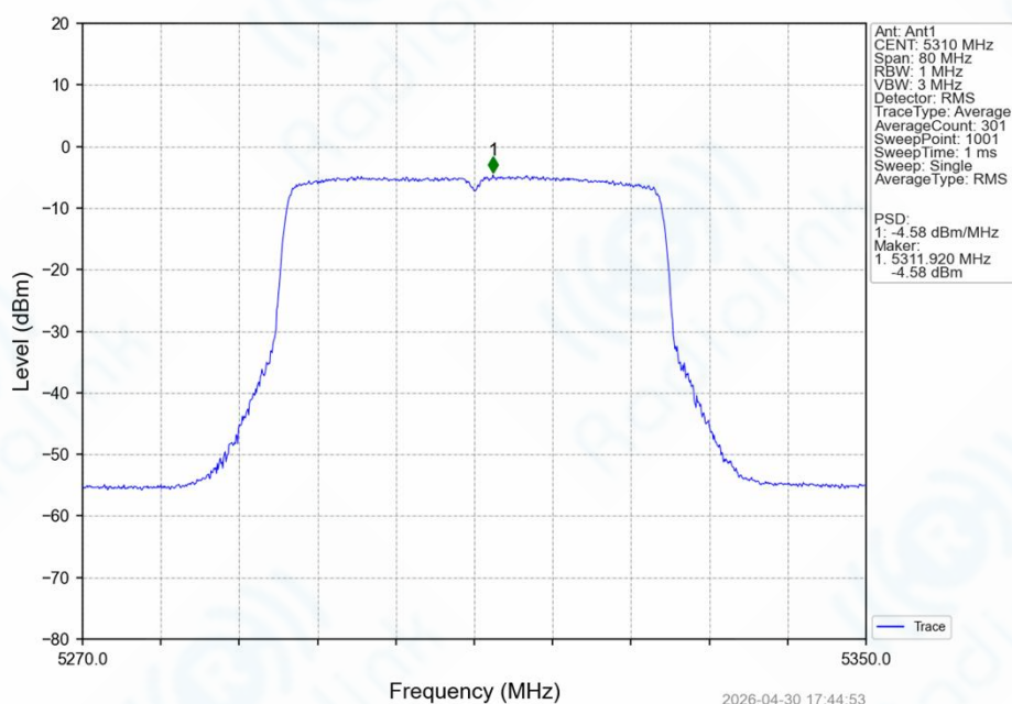
802.11ax(HEW40)_HCH_5310MHz_SU / _Ant1_NTNV
