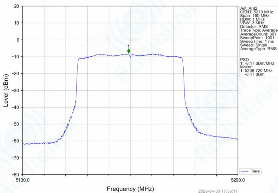
802.11ax(HEW80)_MCH_5210MHz_SU / MIMO_NTNV
