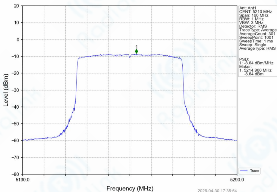
802.11ax(HEW80)_MCH_5210MHz_SU / _Ant1_NTNV
