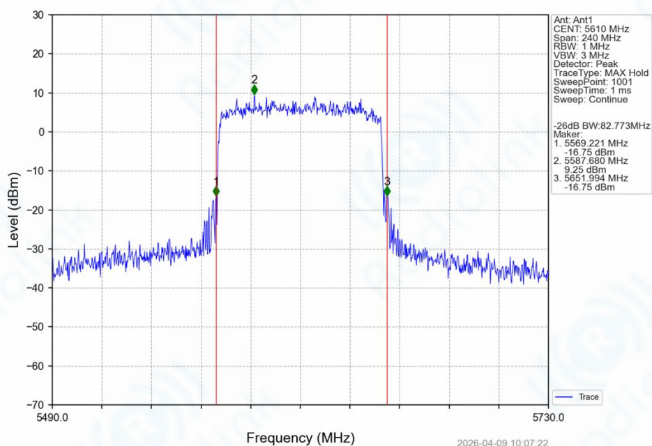
802.11ax(HEW80)_HCH_5610MHz_SU / _Ant1_NTNV
