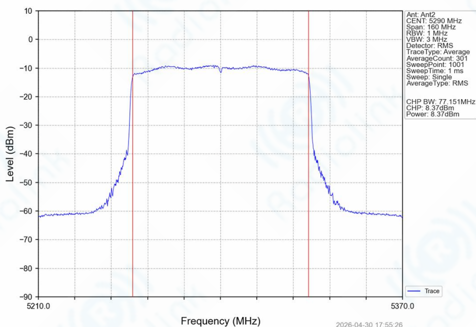
802.11ax(HEW80)_MCH_5290MHz_SU / _Ant2_NTNV
