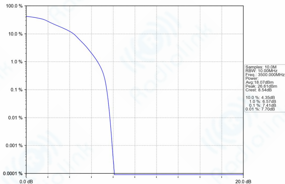
Band42_10MHz_16QAM_MCH_3500MHz_RB_50_0_NTNV
