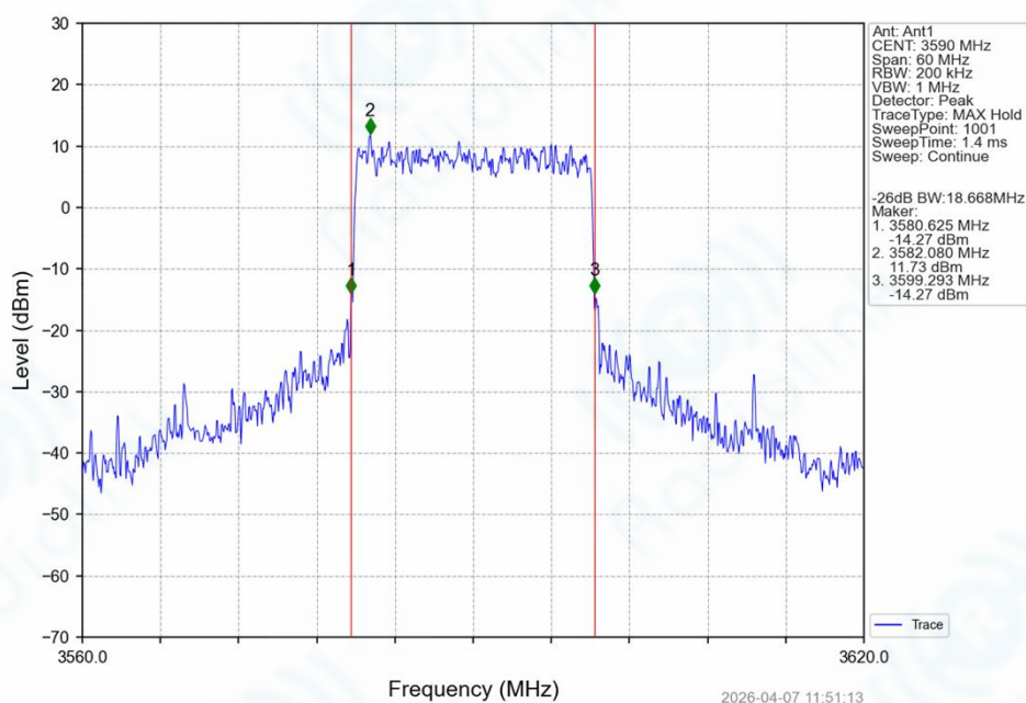
Band42_20MHz_QPSK_HCH_3590MHz_RB_100_0_NTNV
