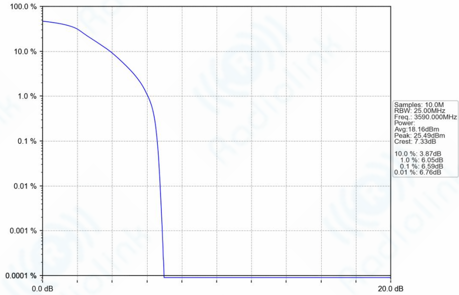
Band42_20MHz_QPSK_HCH_3590MHz_RB_100_0_NTNV
