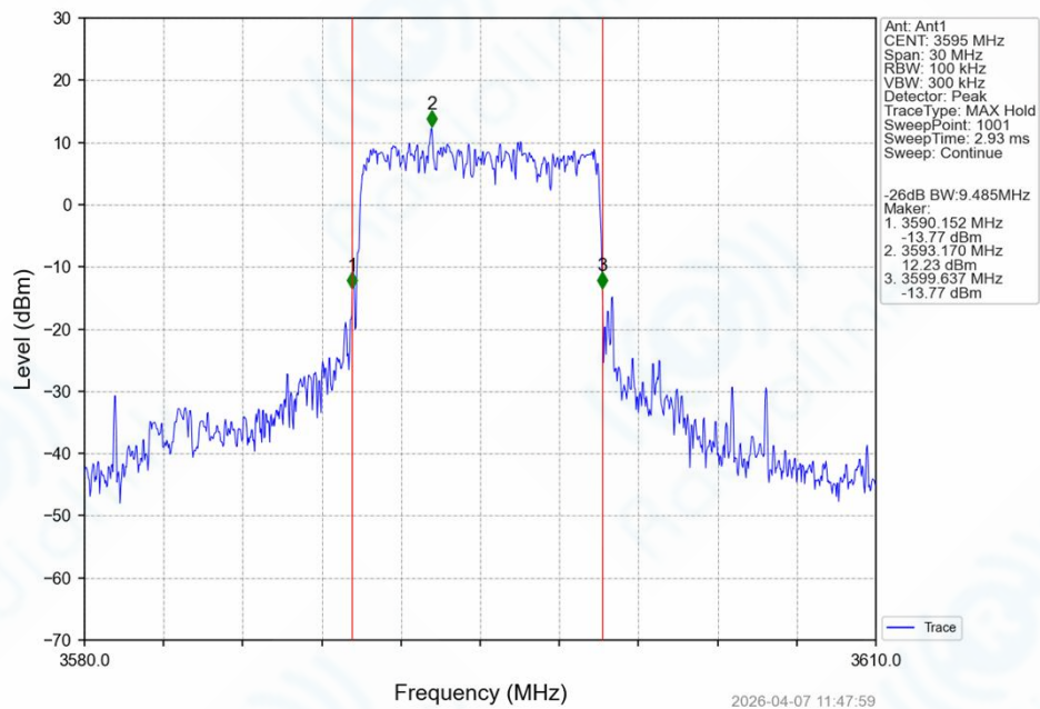
Band42_10MHz_QPSK_HCH_3595MHz_RB_50_0_NTNV
