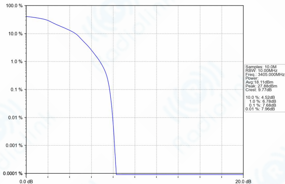
Band42_10MHz_16QAM_LCH_3405MHz_RB_50_0_NTNV
