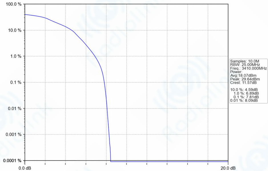
Band42_20MHz_16QAM_LCH_3410MHz_RB_100_0_NTNV
