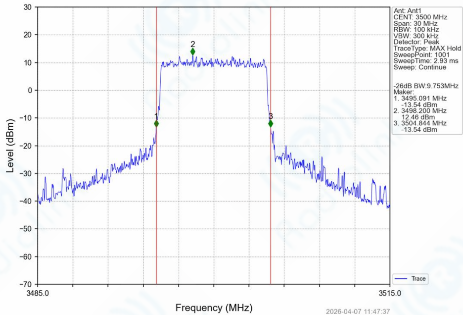
Band42_10MHz_16QAM_MCH_3500MHz_RB_50_0_NTNV
