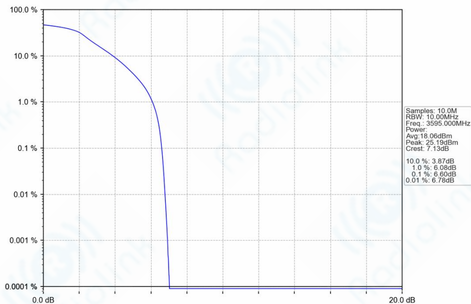
Band42_10MHz_QPSK_HCH_3595MHz_RB_50_0_NTNV
