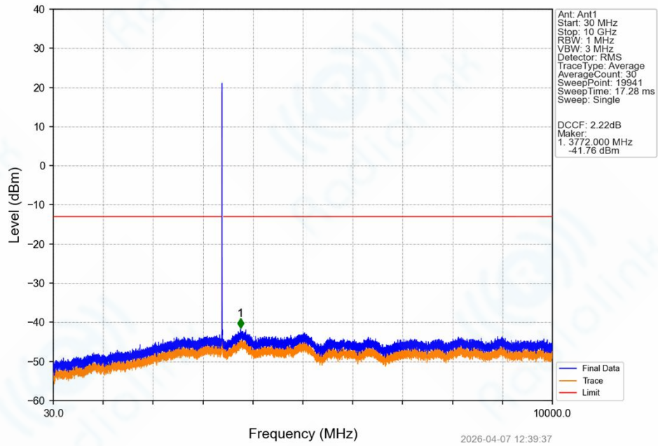
Band42_10MHz_16QAM_LCH_3405MHz_RB_1_0_NTNV
