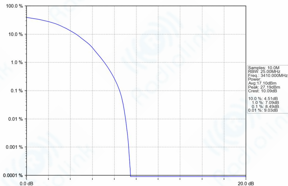
Band42_20MHz_64QAM_LCH_3410MHz_RB_100_0_NTNV
