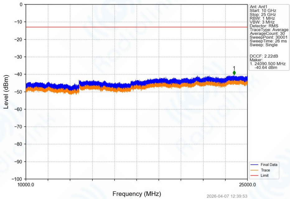
Band42_10MHz_16QAM_LCH_3405MHz_RB_1_0_NTNV
