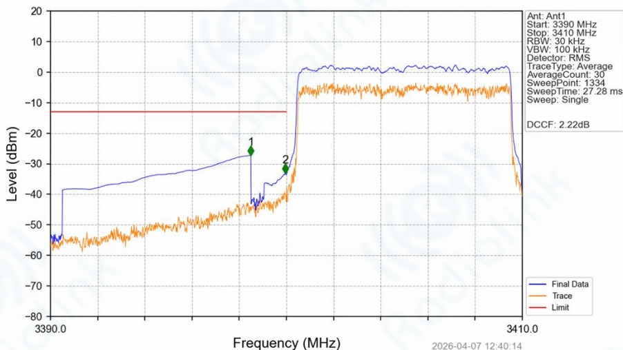
Band42_10MHz_16QAM_LCH_3405MHz_RB_50_0_NTNV
