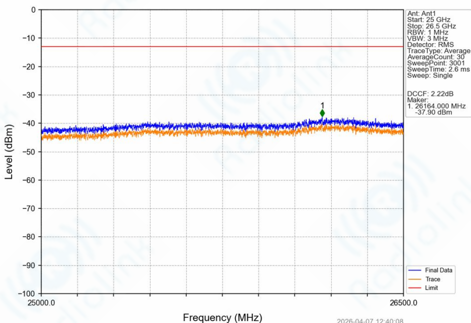
Band42_10MHz_16QAM_LCH_3405MHz_RB_50_0_NTNV
