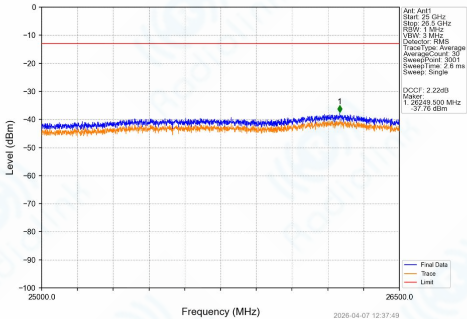
Band42_10MHz_QPSK_LCH_3405MHz_RB_1_0_NTNV
