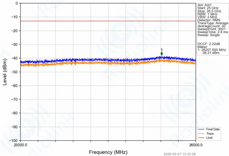
Band42_10MHz_QPSK_HCH_3595MHz_RB_1_49_NTNV
