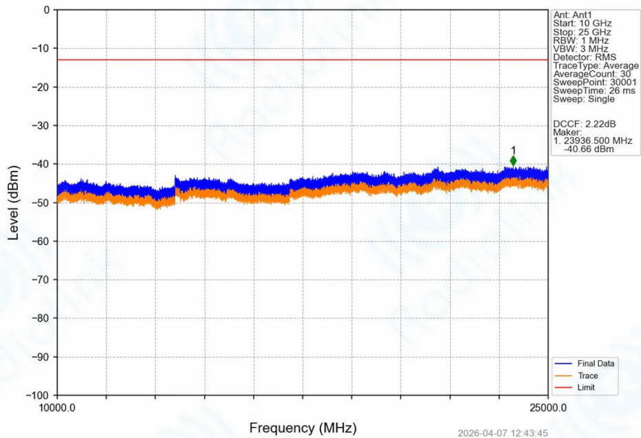
Band42_10MHz_16QAM_MCH_3500MHz_RB_1_0_NTNV
