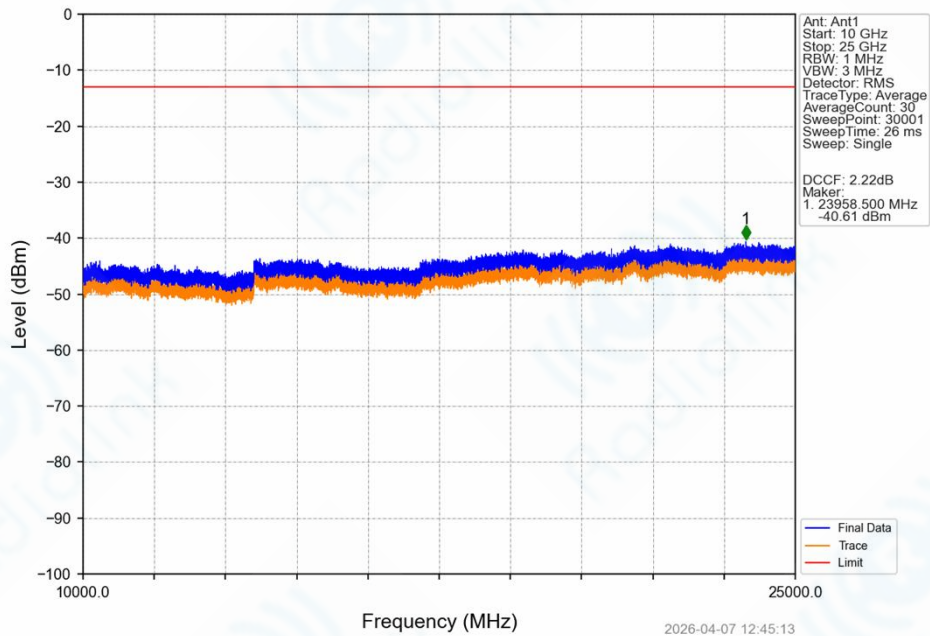
Band42_10MHz_QPSK_HCH_3595MHz_RB_1_0_NTNV
