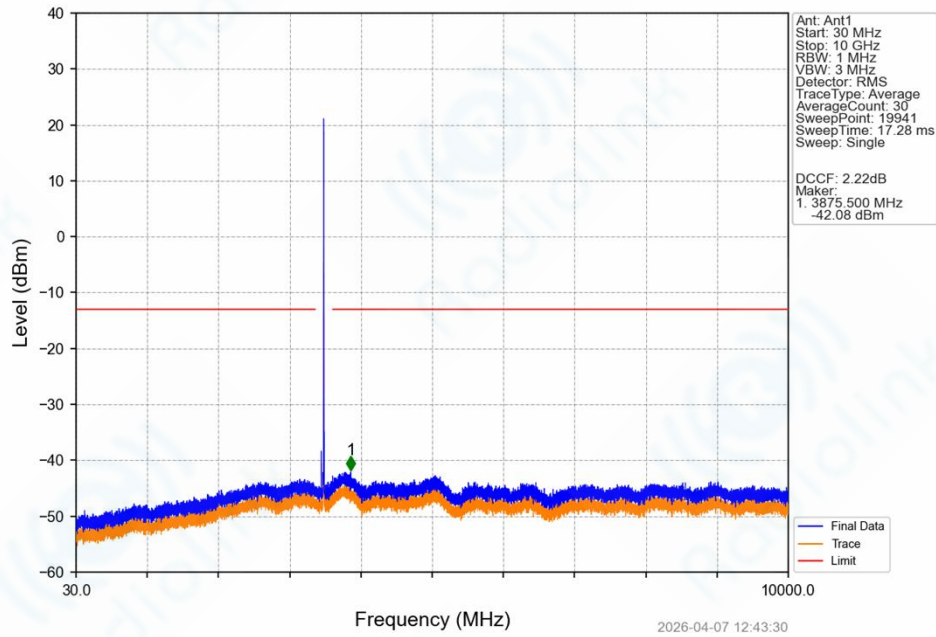
Band42_10MHz_16QAM_MCH_3500MHz_RB_1_0_NTNV
