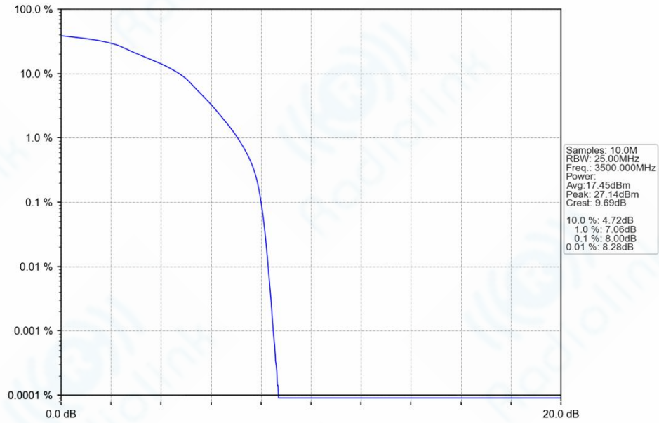
Band42_20MHz_16QAM_MCH_3500MHz_RB_100_0_NTNV
