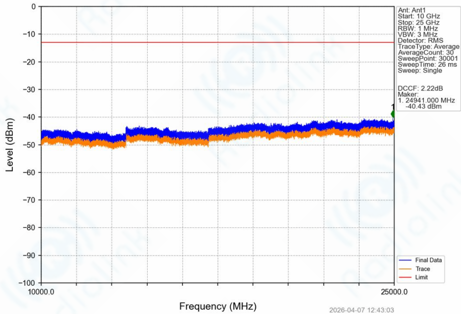
Band42_10MHz_QPSK_MCH_3500MHz_RB_1_0_NTNV
