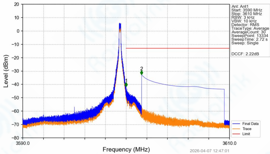
Band42_10MHz_QPSK_HCH_3595MHz_RB_1_49_NTNV
