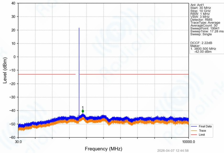
Band42_10MHz_QPSK_HCH_3595MHz_RB_1_0_NTNV
