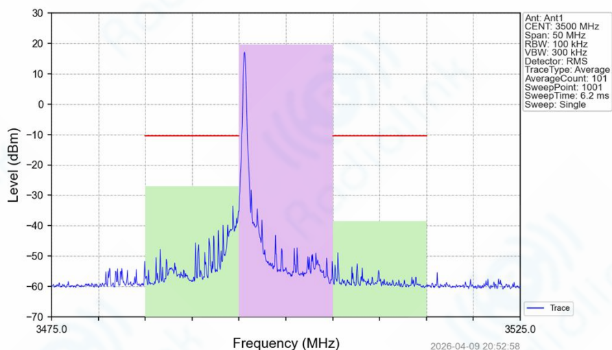
Band42_10MHz_16QAM_MCH_3500MHz_RB_1_0_NTNV
