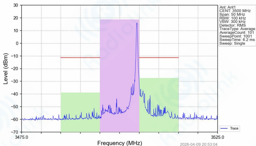
Band42_10MHz_16QAM_MCH_3500MHz_RB_1_49_NTNV
