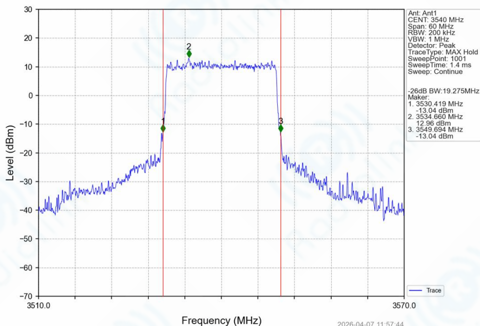
Band42a_20MHz_QPSK_HCH_3540MHz_RB_100_0_NTNV
