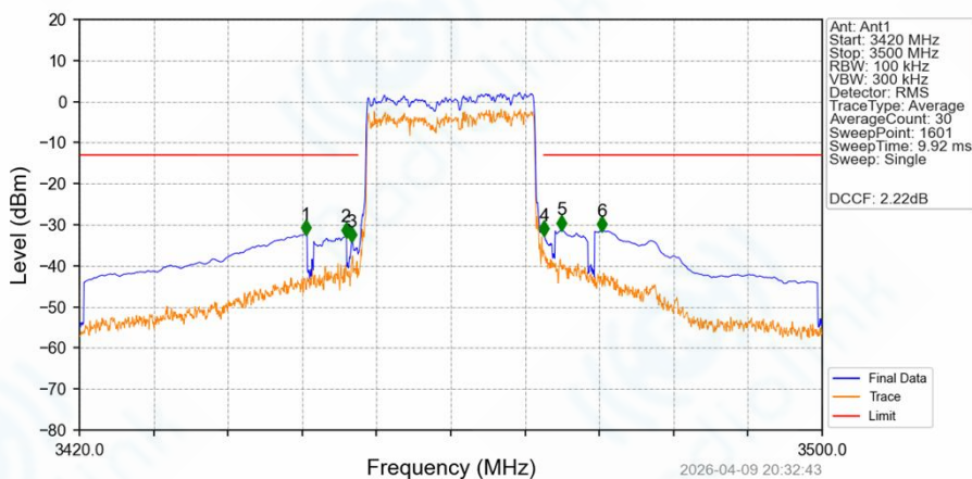
Band42a_20MHz_16QAM_LCH_3460MHz_RB_100_0_NTNV
