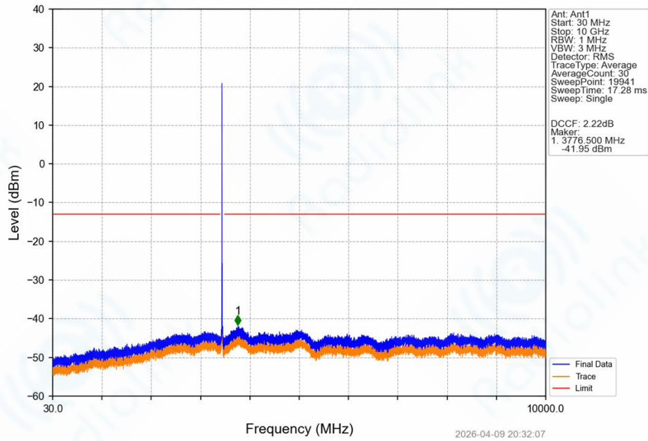
Band42a_20MHz_16QAM_LCH_3460MHz_RB_1_0_NTNV
