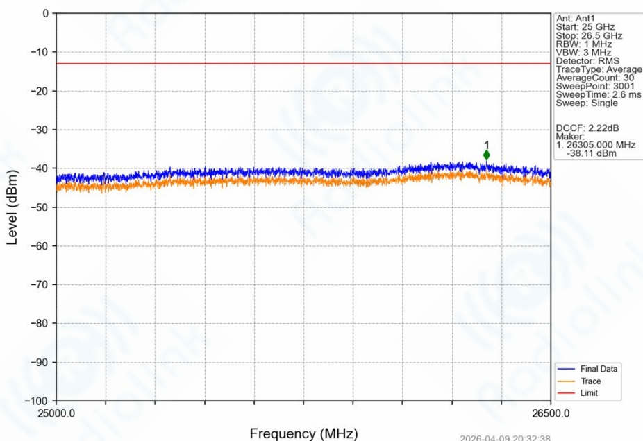
Band42a_20MHz_16QAM_LCH_3460MHz_RB_100_0_NTNV
