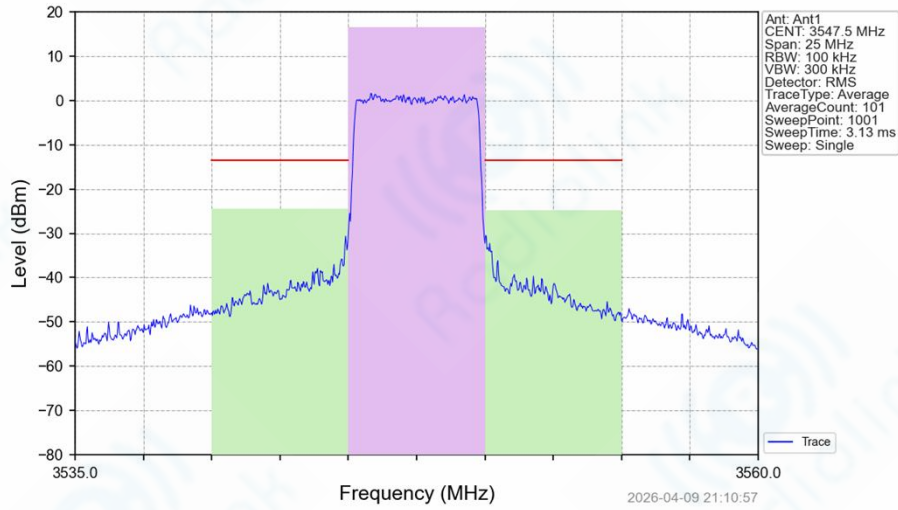
Band42a 5MHz 64QAM HCH 3547.5MHz RB 25 0 NTV
