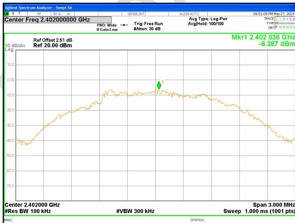
Tx. Spurious NVHT BLE 2M 2402MHz Ant1 Emission
