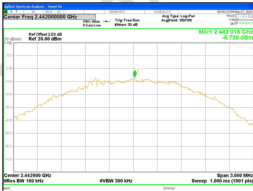
Tx. Spurious NVHT BLE 2M 2442MHz Ant1 Emission
