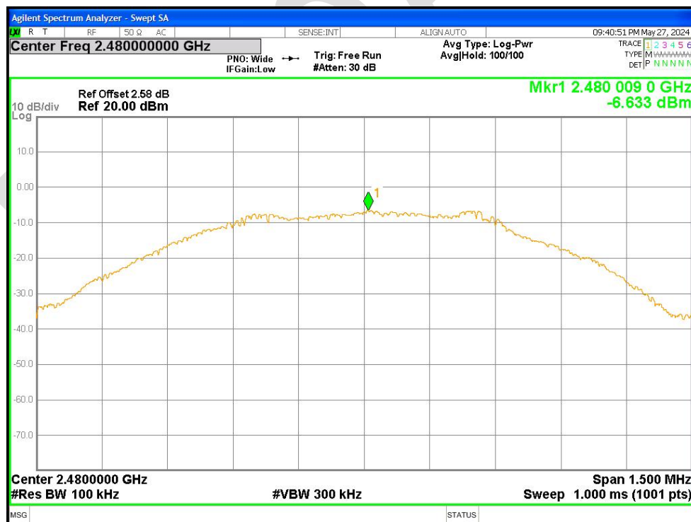
Tx. Spurious NVHT BLE 1M 2480MHz Ant1 Emission
