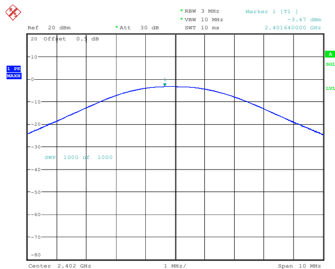
BLE 1Mbps Lowest Channel
