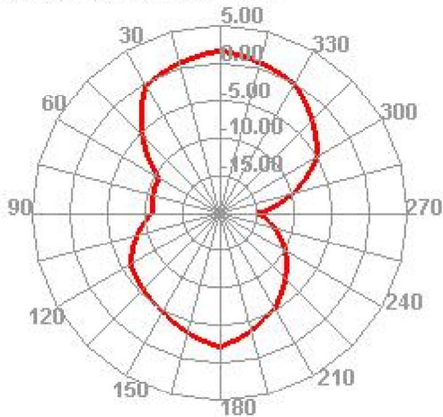
5500.000MHz E1
