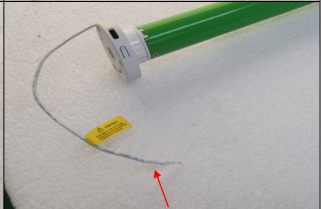
Antenna
