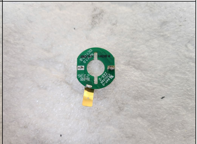
Antenna
