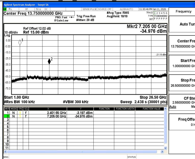
BLE_2M_Ant1_2402_1000~26500
