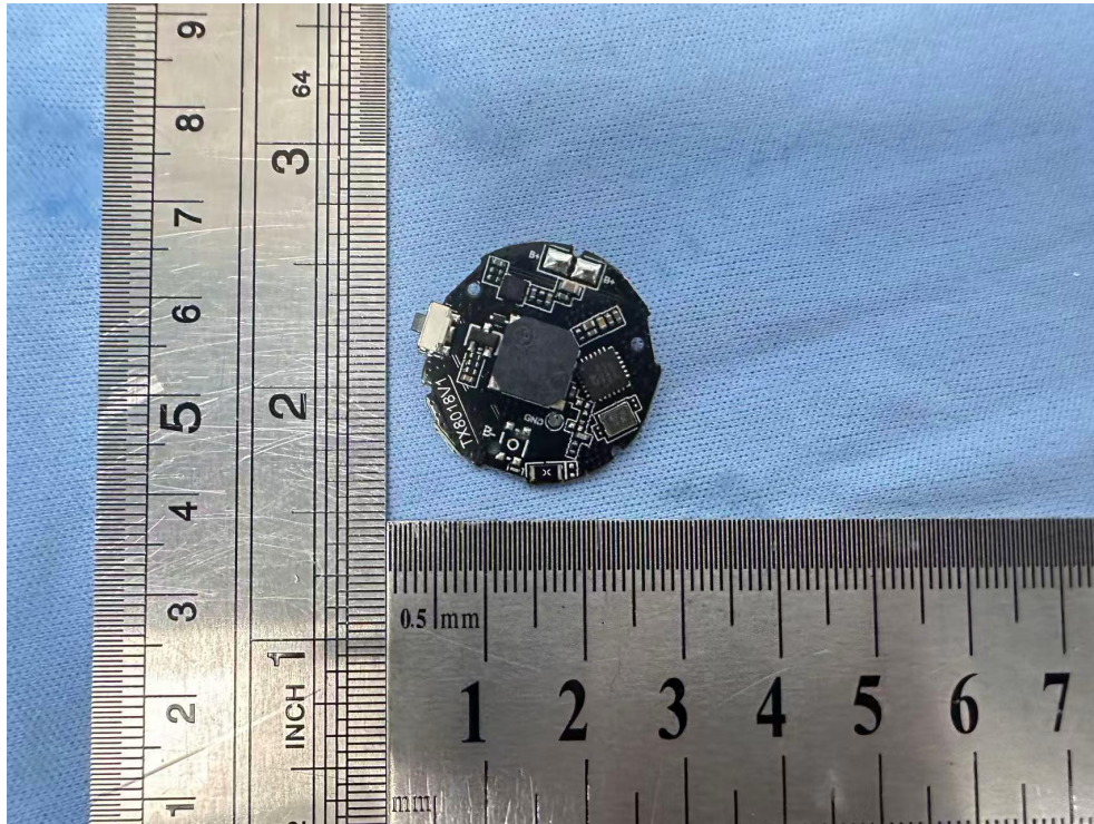
Internal Photos(TX01)
