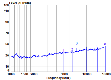
BLE_1M_TX_CH_39_Vertical-Avg
