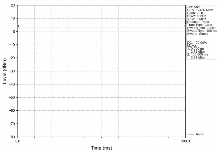
2M_HCH_2480MHz_Ant1_NTNV
