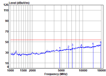
BLE_2M_TX_CH_00_Vertical-Avg
