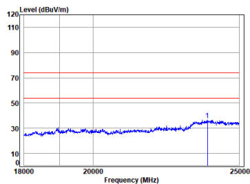
BLE 1M_TX_CH_M_Horizontal
