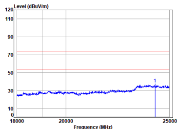
BLE 2M_TX_CH_M_Horizontal
