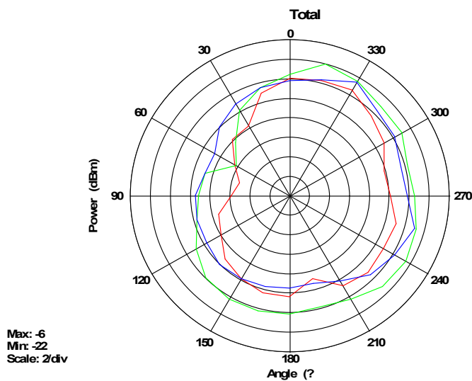
Free Space (WIRPAS NRF52832)
