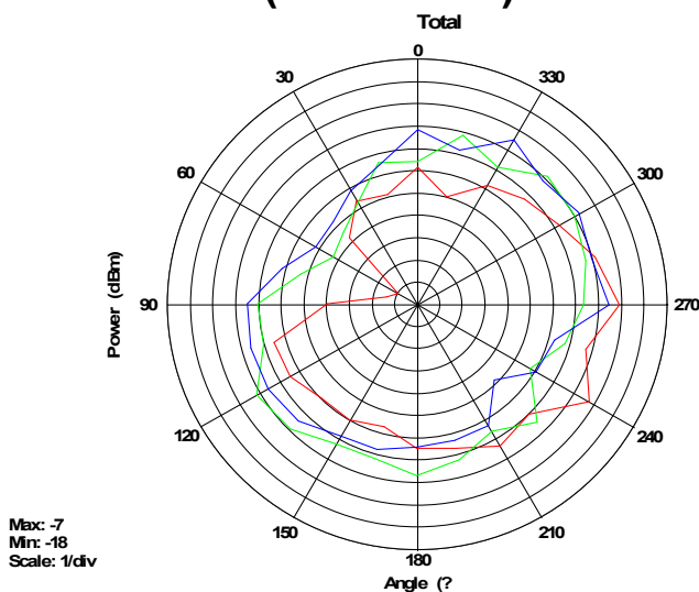
Free Space (BLE NRF52840)
