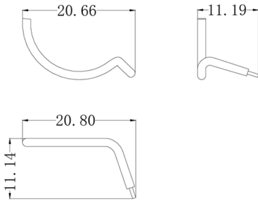
Antenna Dimensions (BLE NRF52840 & WIRPAS NRF52832)
