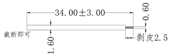
天线展平视图
