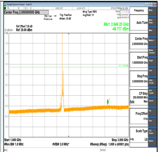
Band2-20MHz-QPSK-19100-1RB#0-1000~3000-PASS
