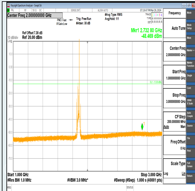
Band2-20MHz-QPSK-18900-1RB#99-1000~3000-PASS
