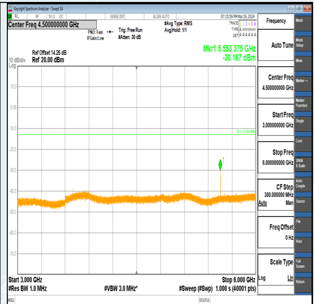
Band2-20MHz-QPSK-18700-1RB#0-3000~6000-PASS
