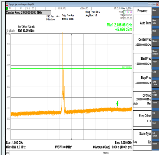
Band2-20MHz-QPSK-18700-1RB#0-1000~3000-PASS
