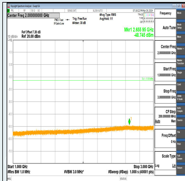
Band2-20MHz-QPSK-18900-1RB#0-1000~3000-PASS
