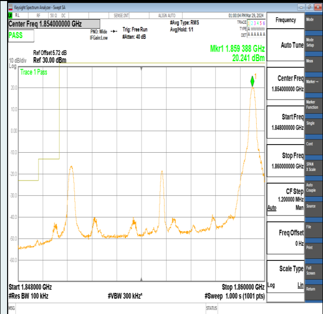
Band2-10MHz-QPSK-18650-1RB#49-PASS
