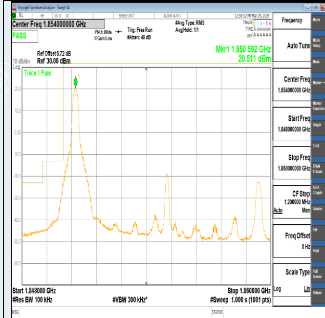
Band2-10MHz-QPSK-18650-1RB#0-PASS
