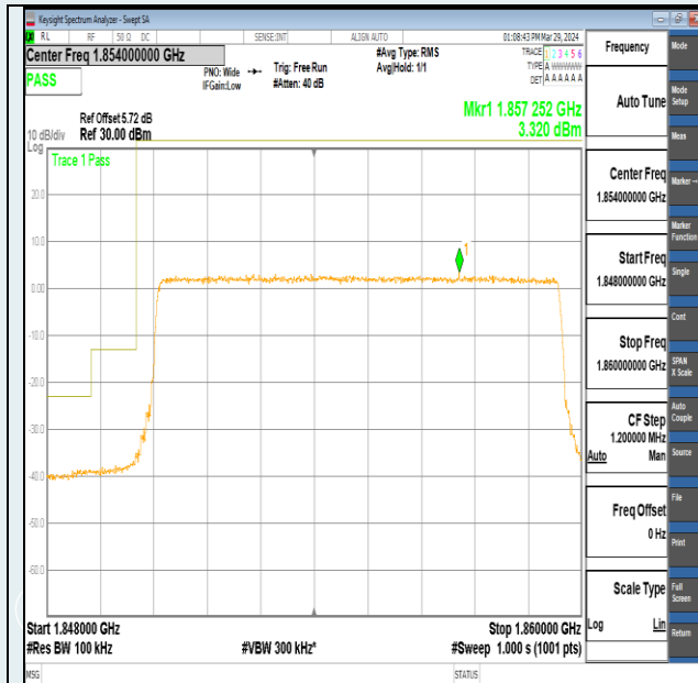
Band2-10MHz-QPSK-18650-50RB#0-PASS
