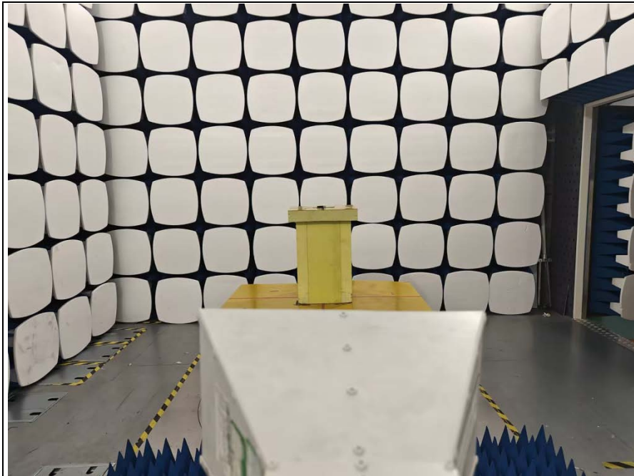
RSE 1GHz-18GHz
