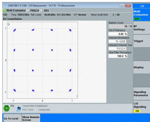
Band2-20MHz-16QAM-19100-100RB#0
