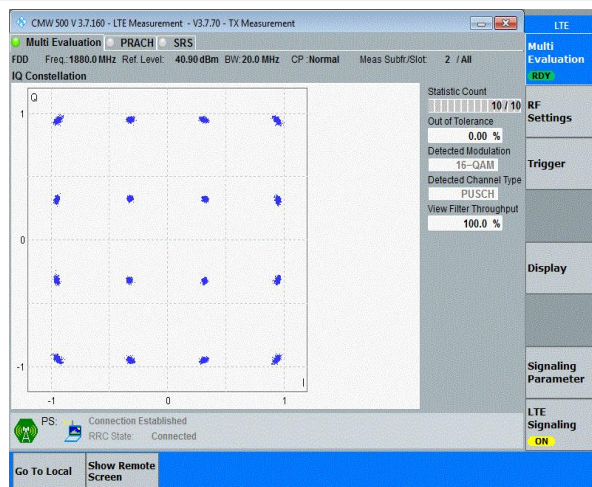
Band2-20MHz-16QAM-19100-100RB#0
