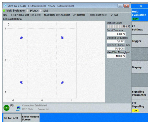
Band2-20MHz-QPSK-19100-100RB#0
