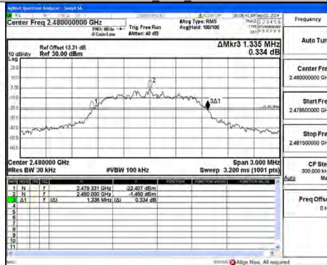
2DH5_Ant1_2480
