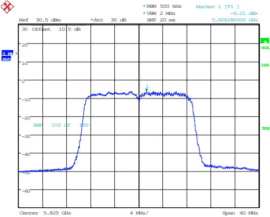
802.11ac20_5825MHz_Chain 0
