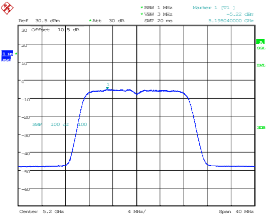
802.11ac20_5200MHz_Chain 1
