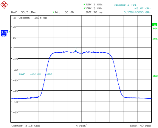
802.11ac20_5180MHz_Chain 0
