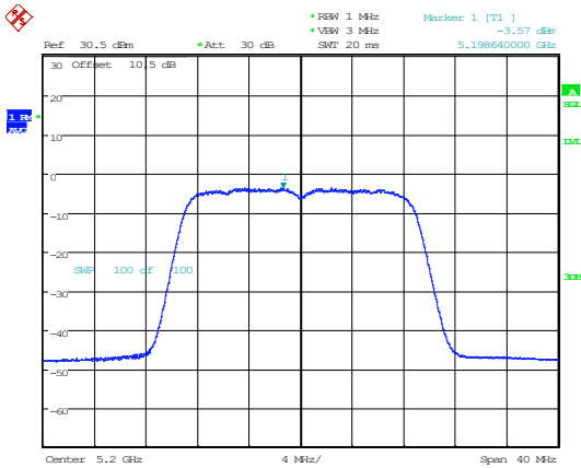
802.11ac20_5200MHz_Chain 0
