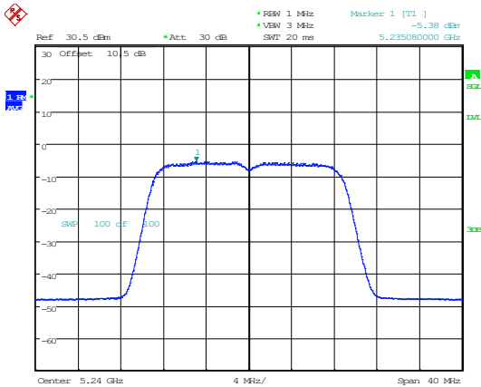
802.11ac20_5240MHz_Chain 1
