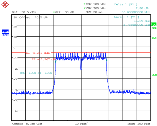
802.11ac40_5755MHz_Chain 0
