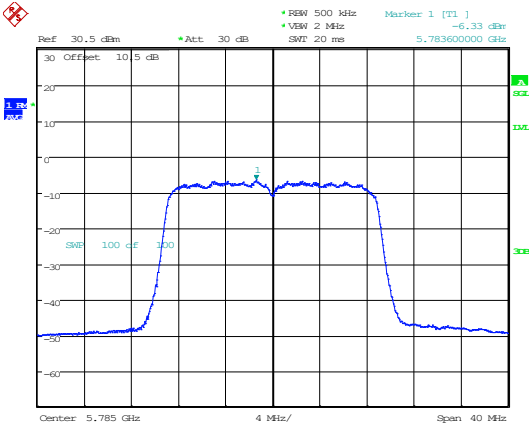
802.11ac20_5785MHz_Chain 0
