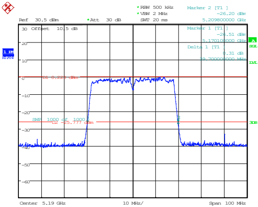
802.11ac40_5190MHz_Chain 0
