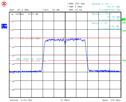
802.11ac40_5230MHz_Chain 0
