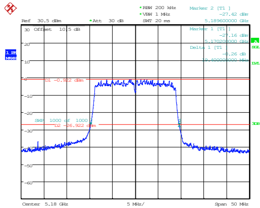
802.11ac20_5180MHz_Chain 0
