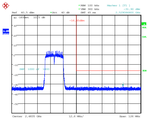
802.11n20_2462MHz_Chain 0
