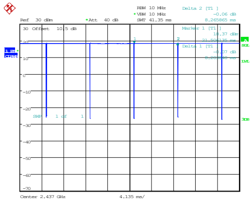
802.11b_2437MHz_Chain 0
