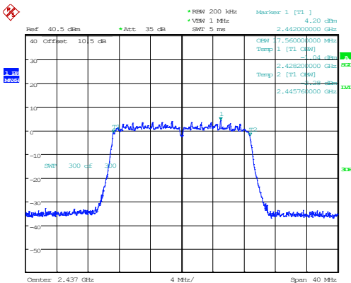
802.11n20_2437MHz_Chain 1
