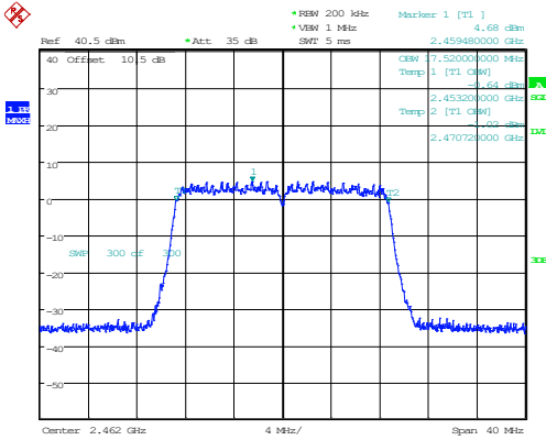
802.11n20_2462MHz_Chain 0
