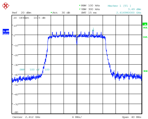
802.11n20_2412MHz_Chain 1
