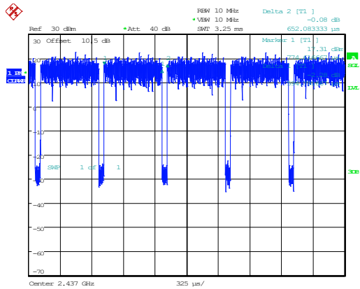
802.11n20_2437MHz_Chain 0
