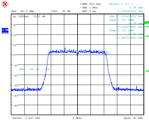
802.11n20_2437MHz_Chain 0
