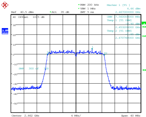
802.11n20_2462MHz_Chain 1
