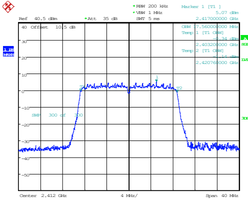
802.11n20_2412MHz_Chain 1
