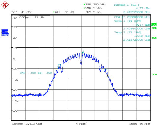
802.11b_2412MHz
