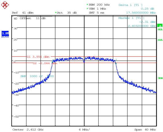
802.11n20_2412MHz
