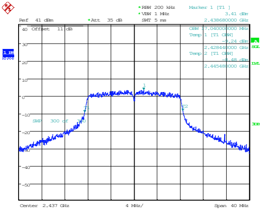
802.11g_2437MHz
