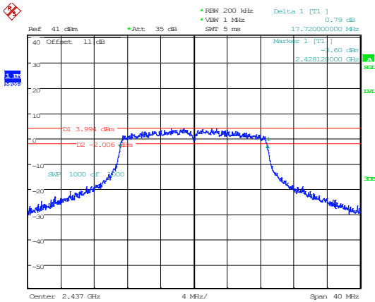
802.11n20_2437MHz
