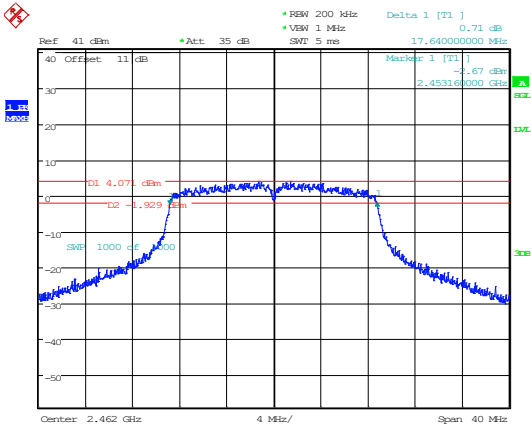
802.11n20_2462MHz
