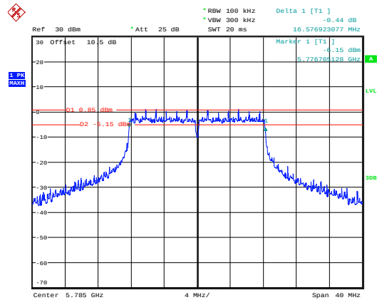
802.11 a_5785MHz
