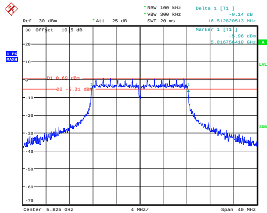
802.11 a_5825MHz
