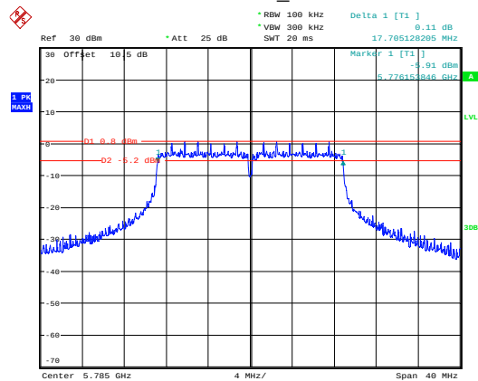
802.11 n20_5785MHz
