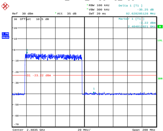
3EDR_DH1_Hopping_Upper
