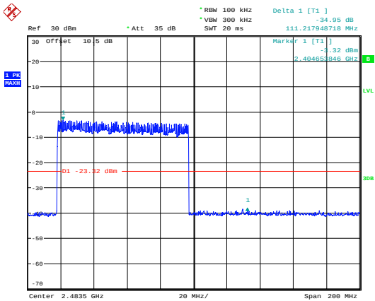
2EDR_DH1_Hopping_Upper
