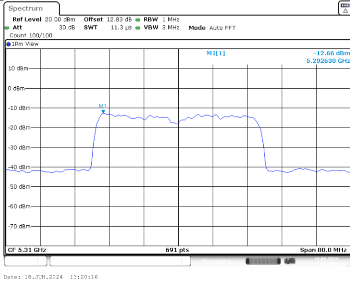
11AX40MIMO_Ant2_5310
