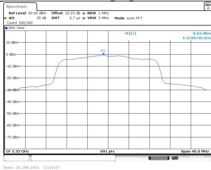
11AX20MIMO_Ant2_5320
