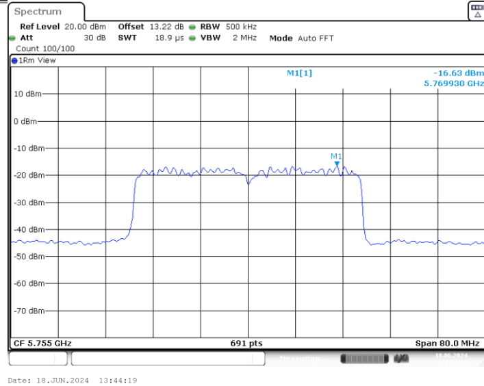
11AX40MIMO_Ant2_5755
