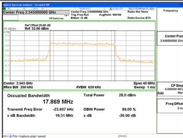
B41(2535-2655) / 20MHz / 16QAM/ Low CH
