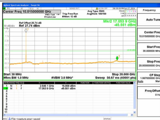
B41(2535-2655)-30M-20G / 10MHz / High CH / QPSK
