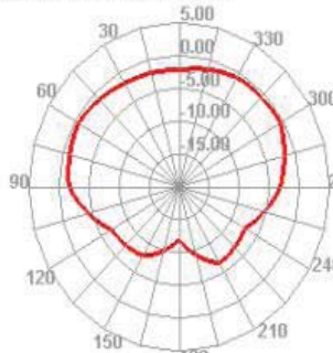
2500.000MHz E1
