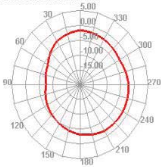
2500.000MHz H
